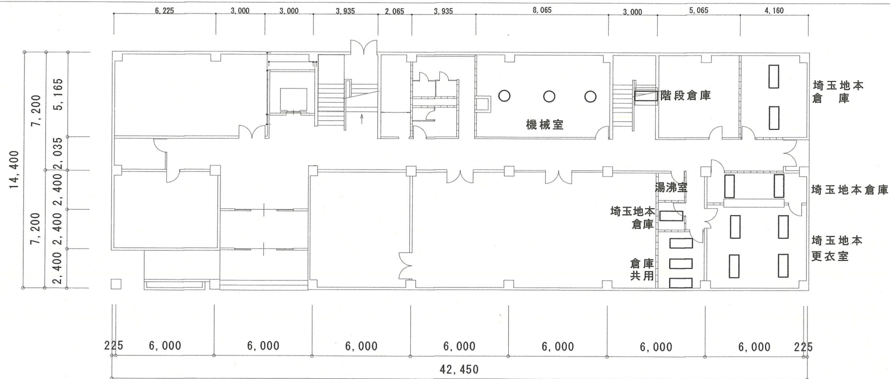
浦和合同庁舎 1号棟 1階平面図
