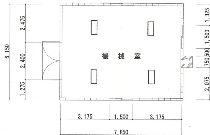
浦和合同庁舎 4号建物平面図
