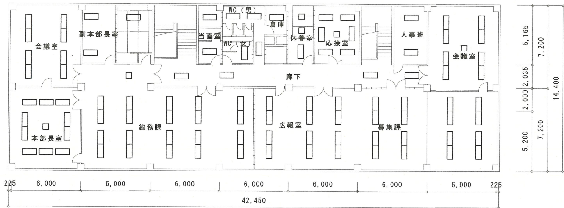
浦和合同庁舎 1号棟 3階平面図
