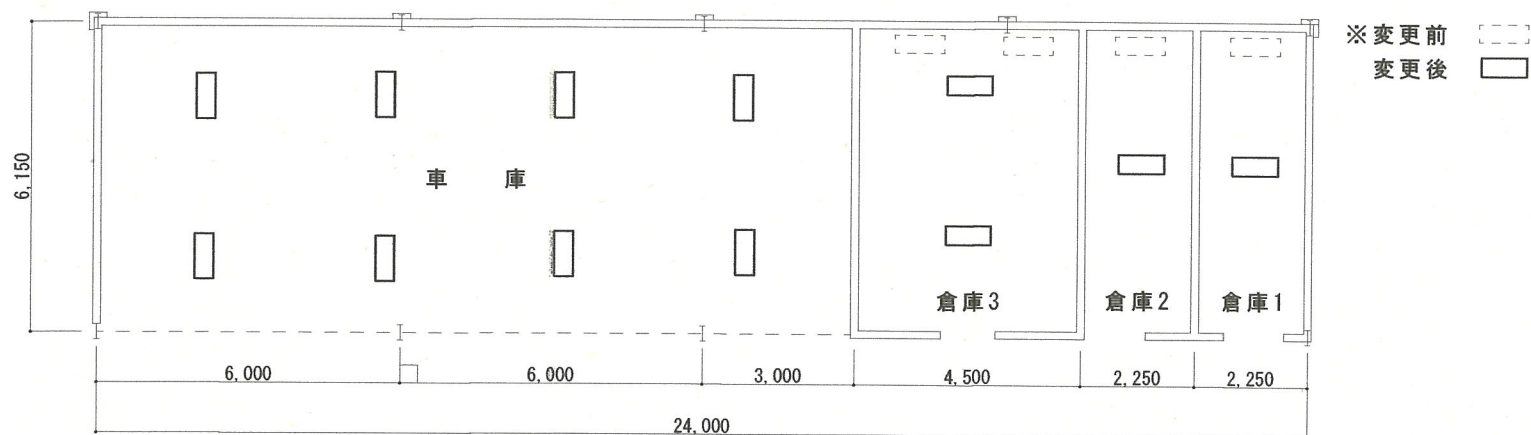
浦和合同庁舎 2号建物平面図
