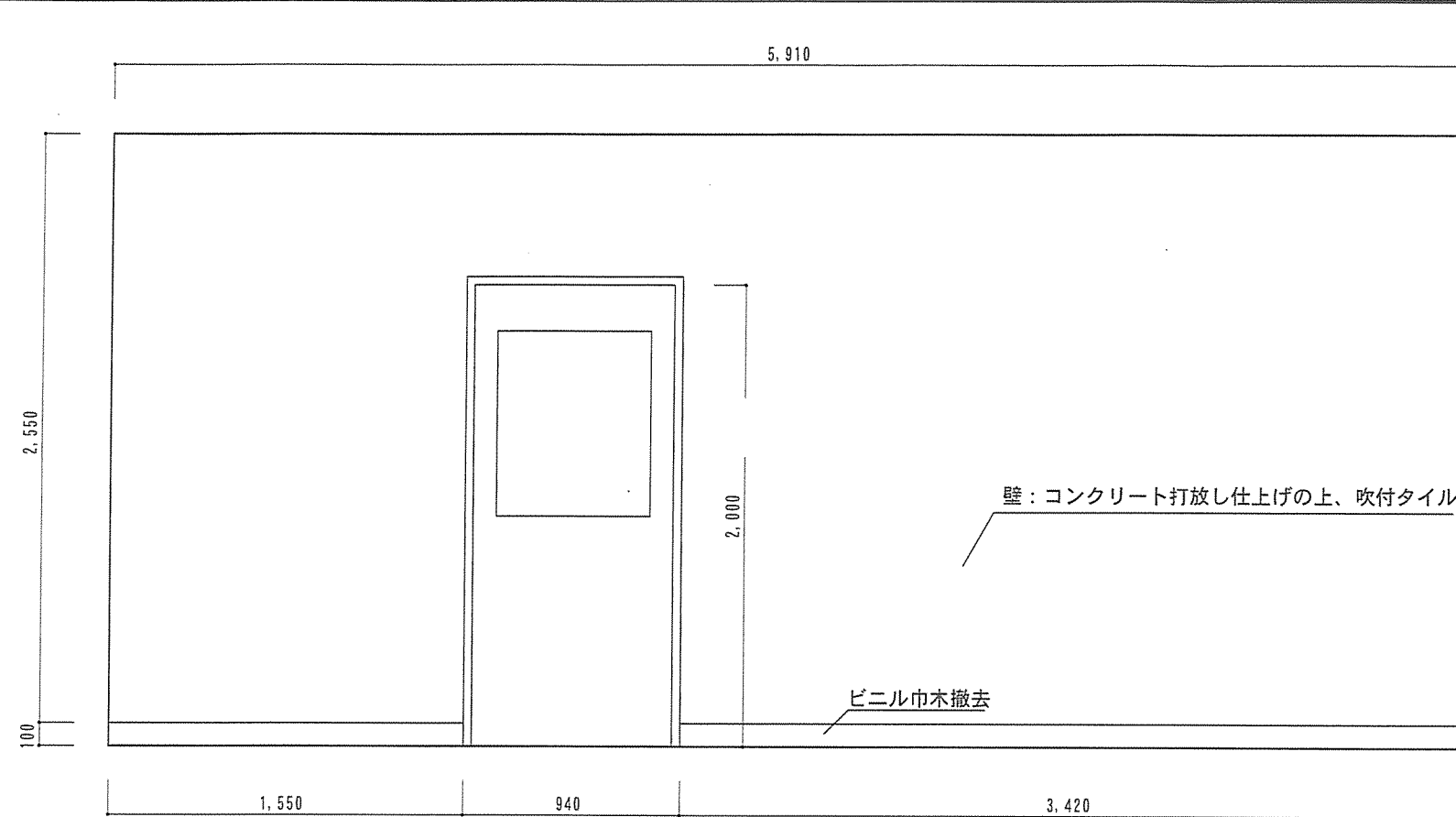
A面展開図 S=1/30 (整備前)
