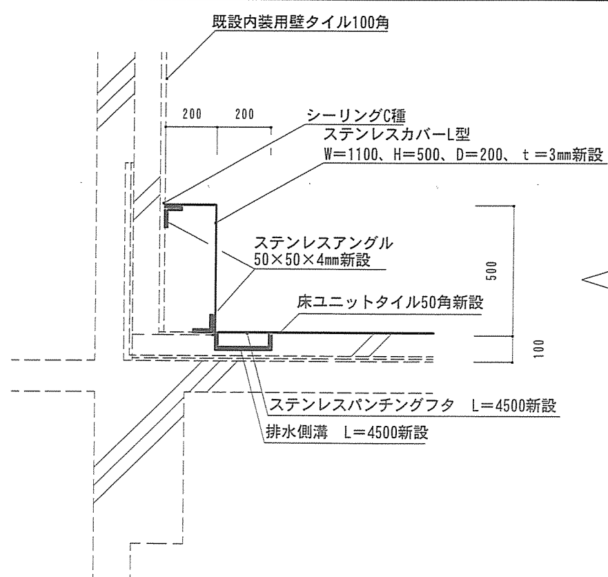
カラバック（B）・排水溝詳細図(整備後) S=1/20
