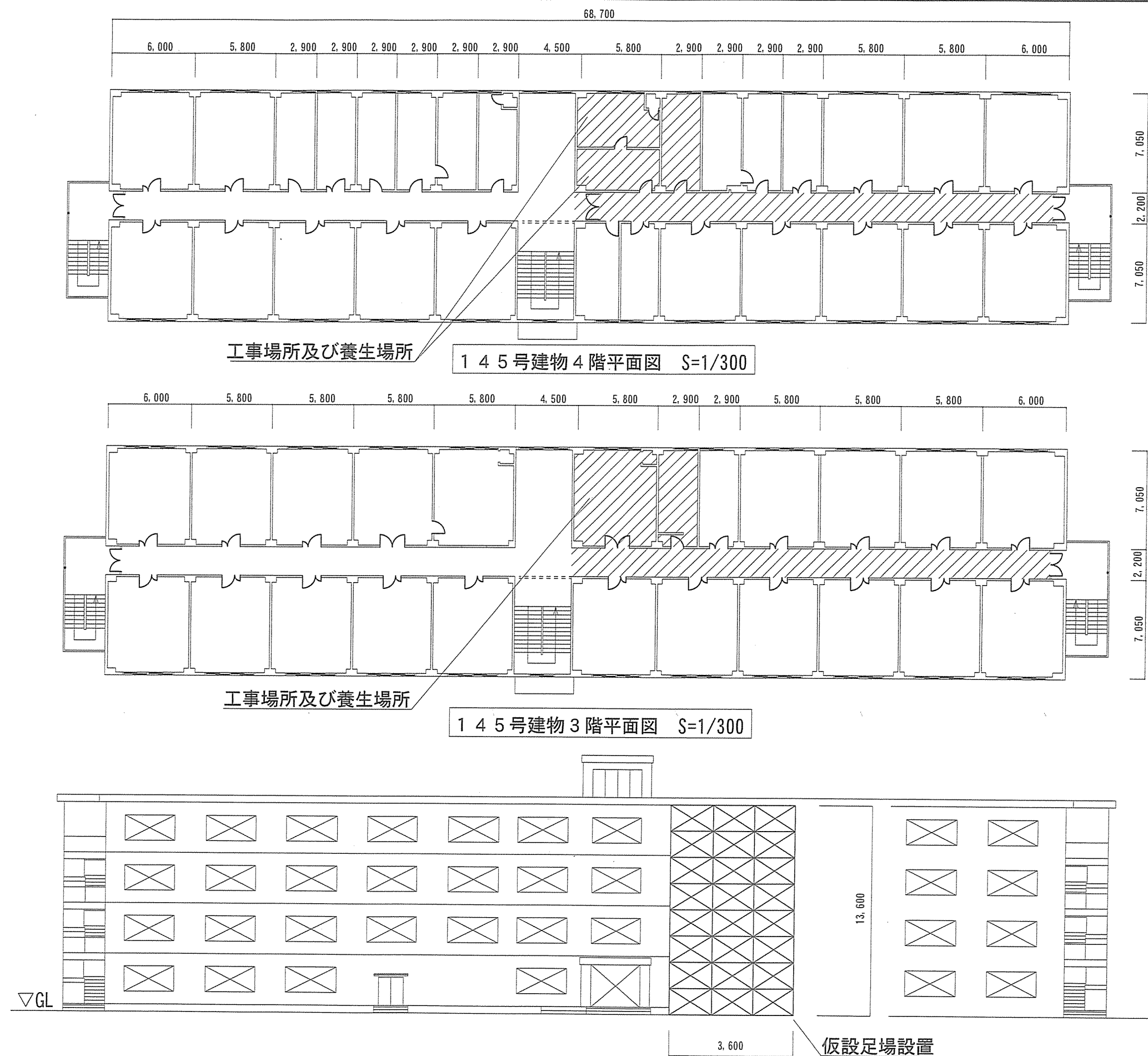
1 4 5 号建物立面図 S=1/300
