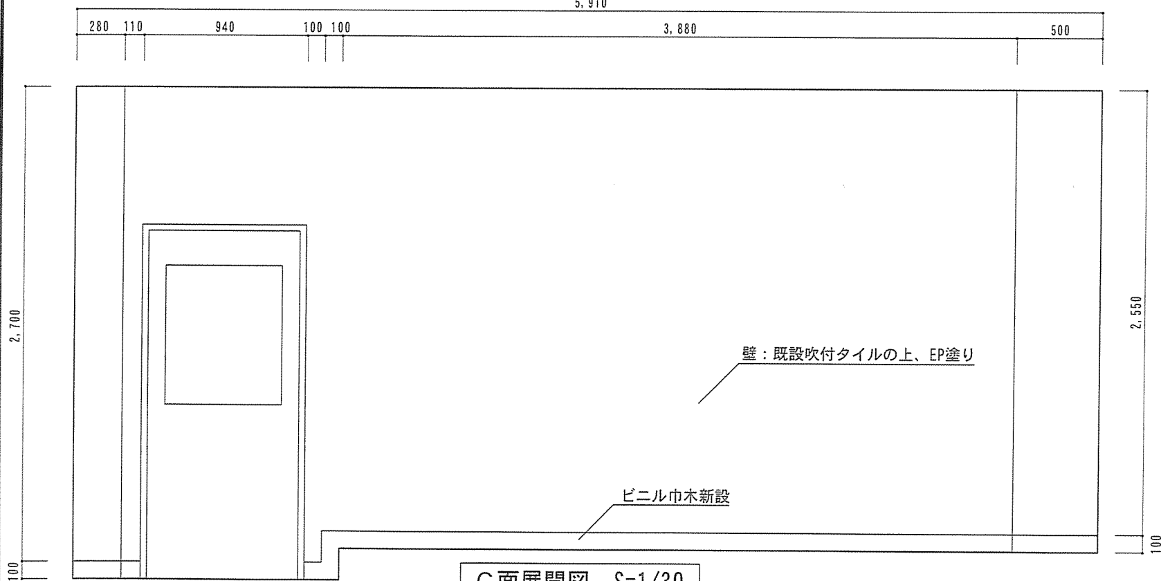
C面展開図 S=1/30 (整備後)
