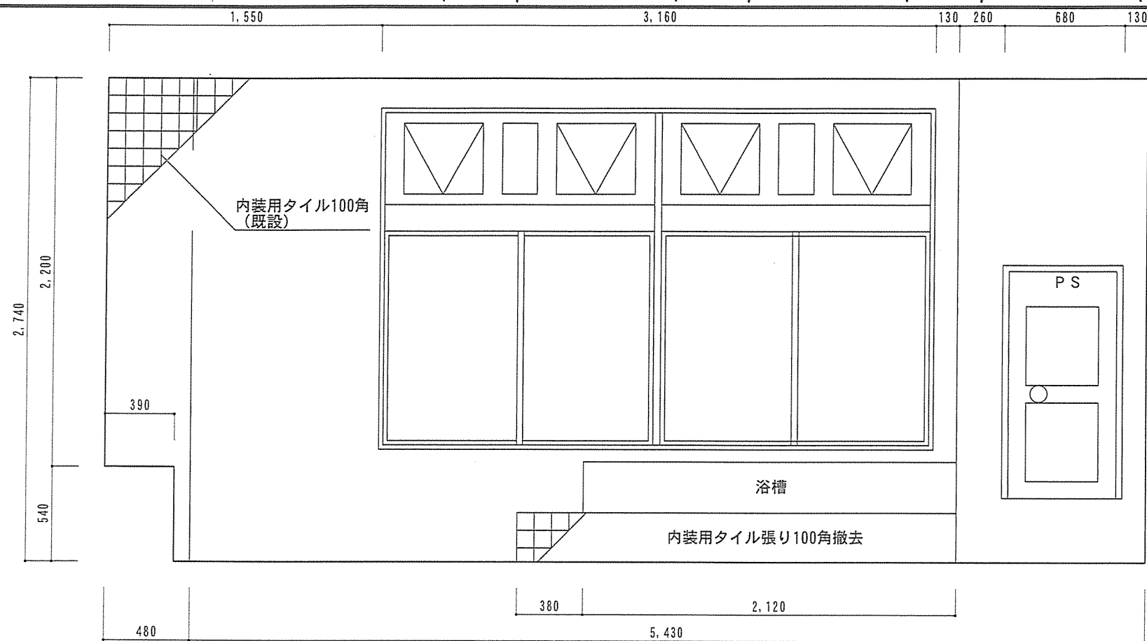
A面展開図 S=1/30 (整備前)
