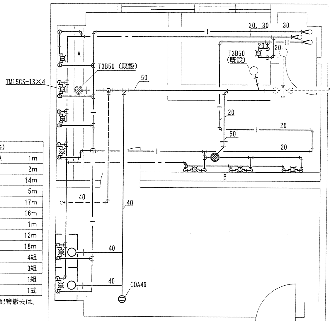
浴室・脱衣所給排水設備図(整備後) S=1/50
