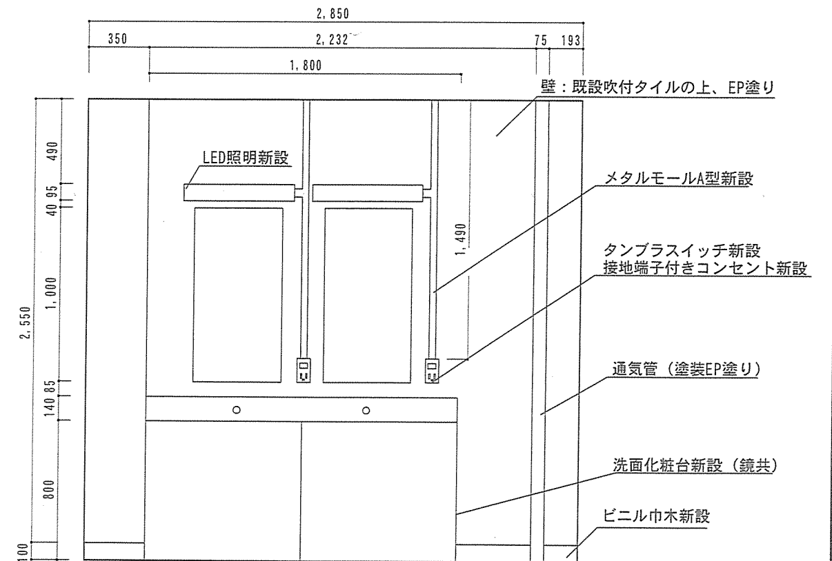
D面展開図 S=1/30 (整備後)
