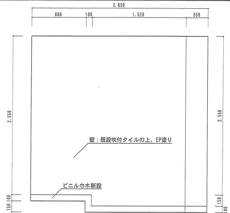
B面展開図 S=1/30 (整備後)
