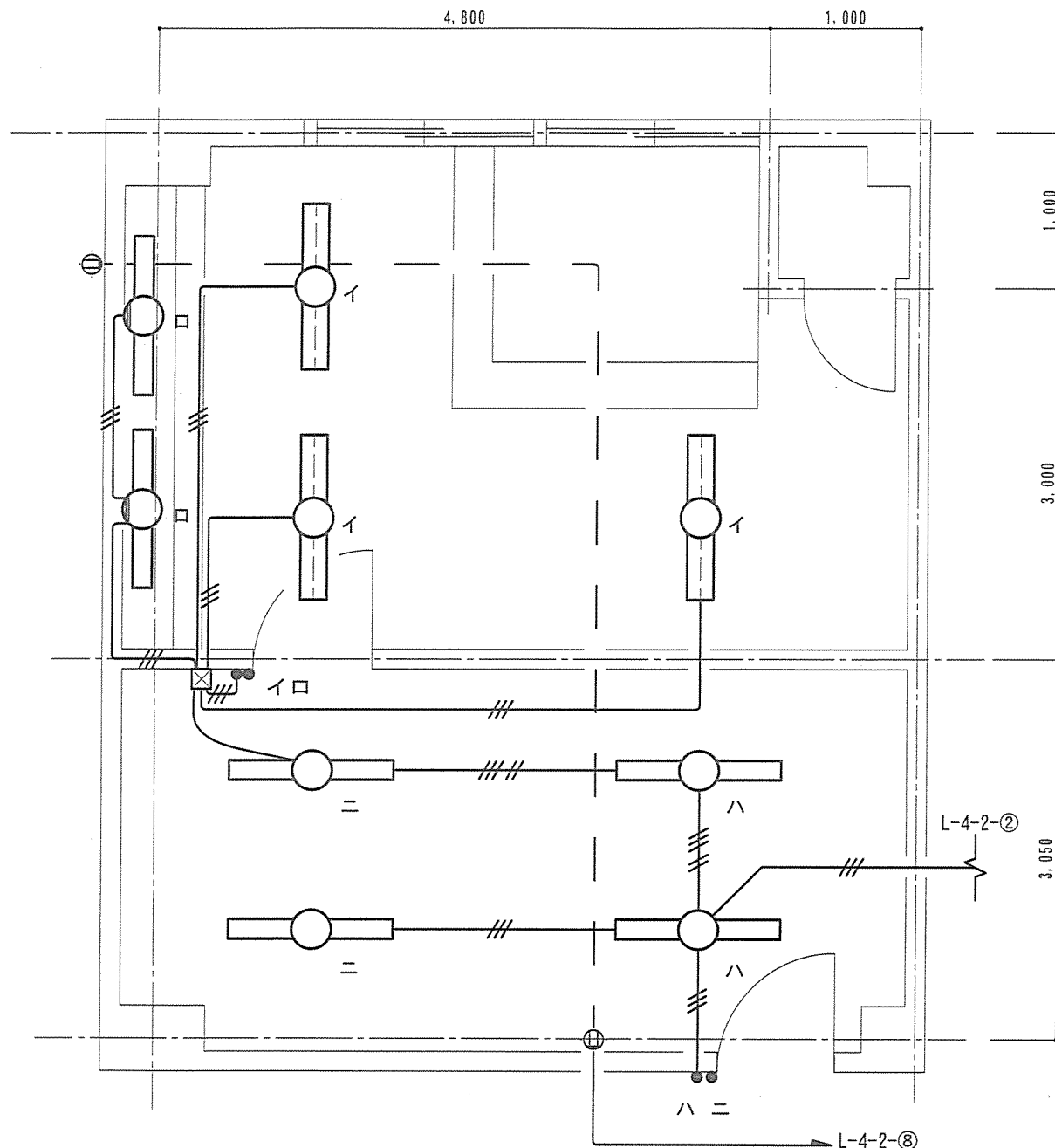
浴室・脱衣所電灯設備図 S=1/50
