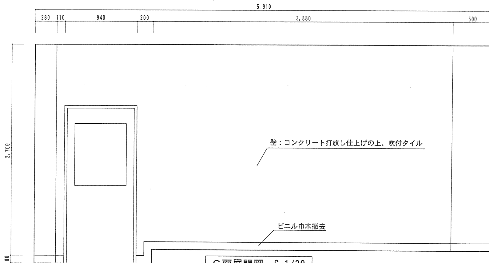
C面展開図 S=1/30 (整備前)
