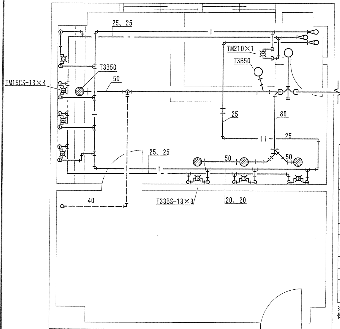
浴室・脱衣所給排水設備図(整備前) S=1/50
