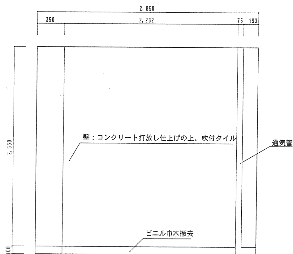
D面展開図 S=1/30 (整備前)
