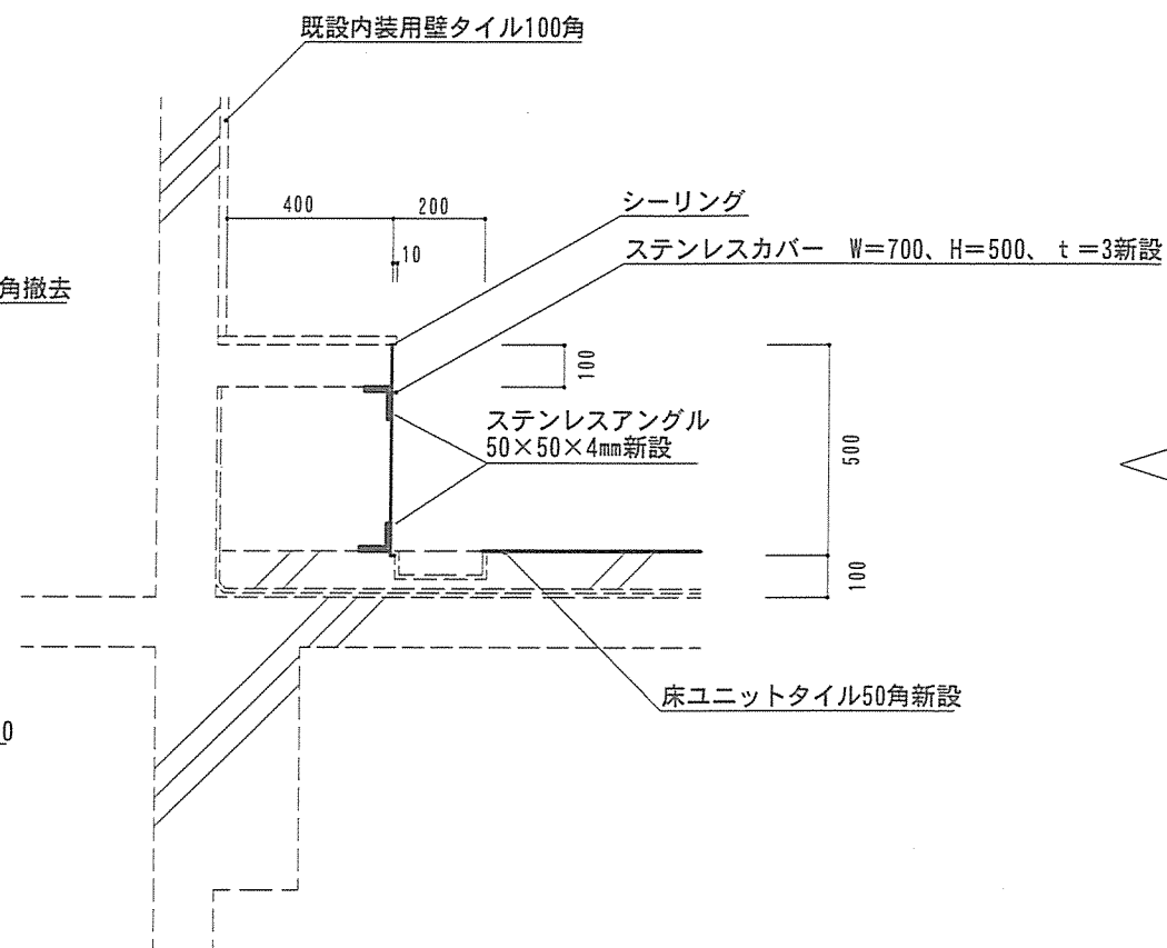
カラバック（A）・排水溝詳細図(整備後) S=1/20
