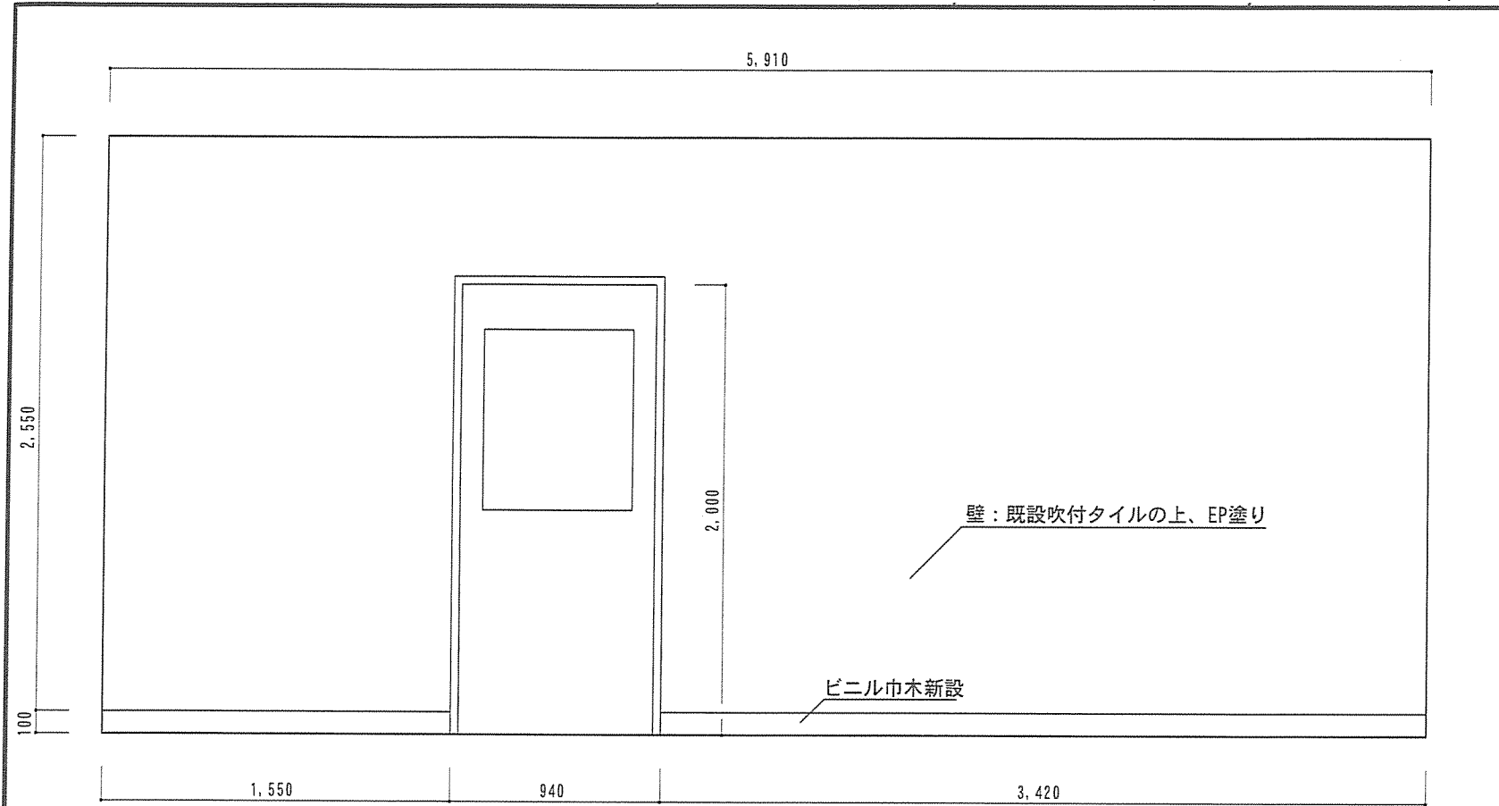
A面展開図 S=1/30 (整備後)
