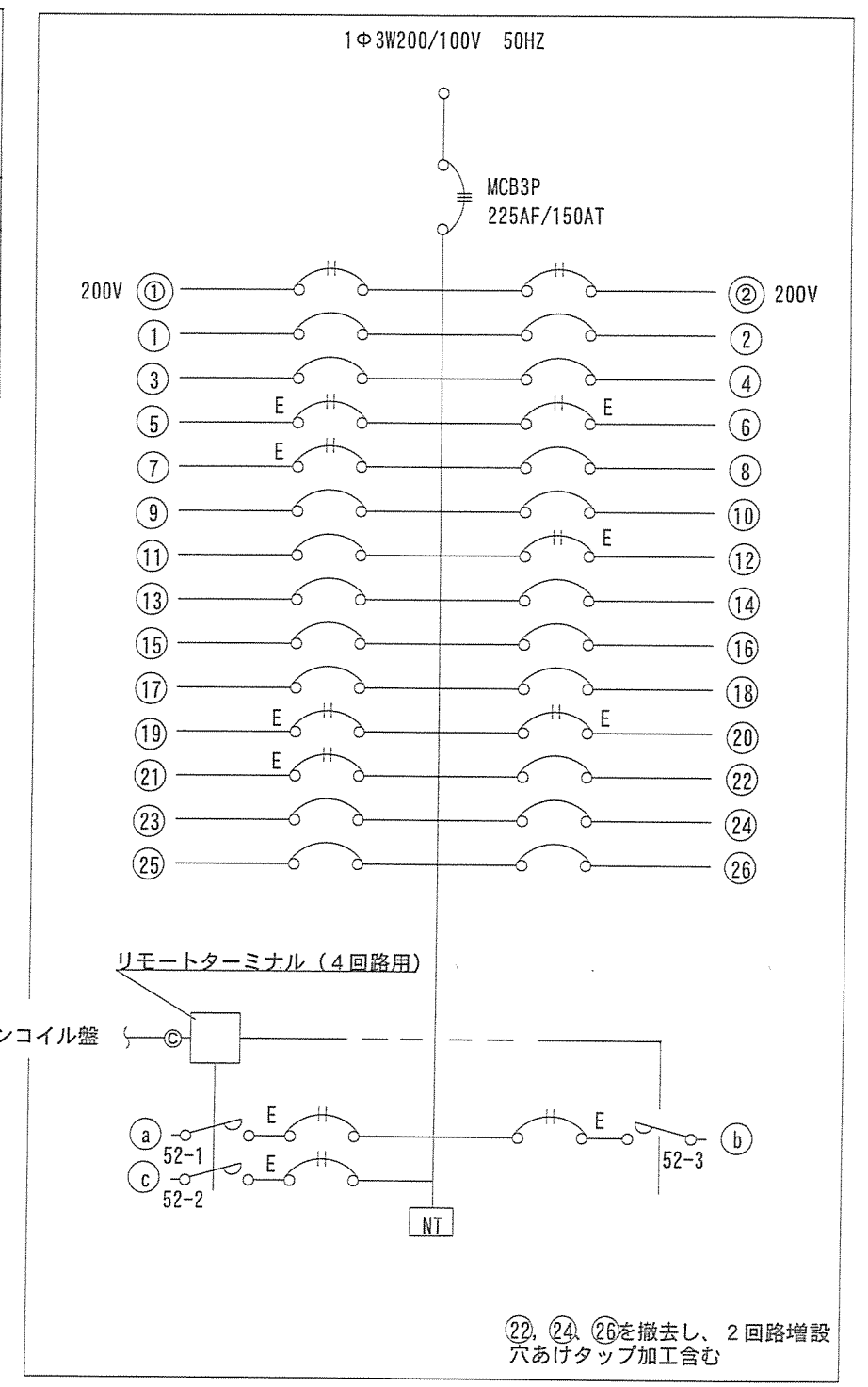
電灯盤結線図 S=1/X
