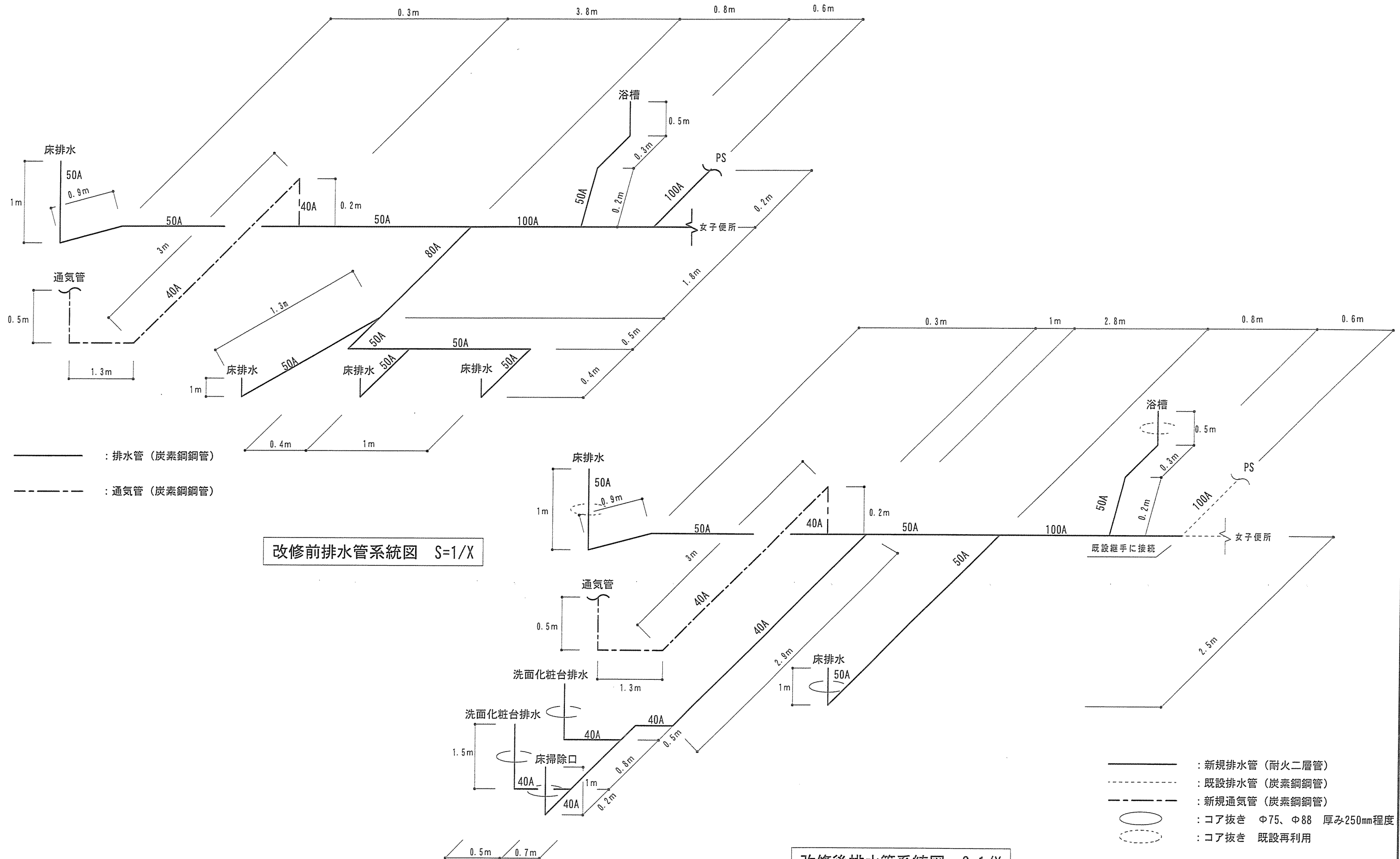
改修後排水系統図 S=1/X
