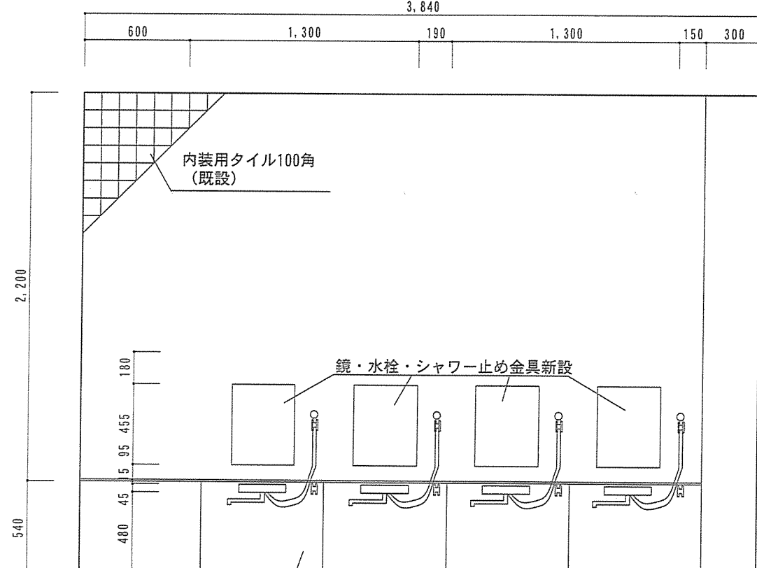
D面展開図 S=1/30 (整備後)
