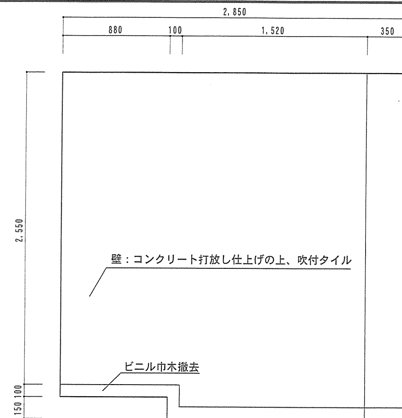
B面展開図 S=1/30 (整備前)
