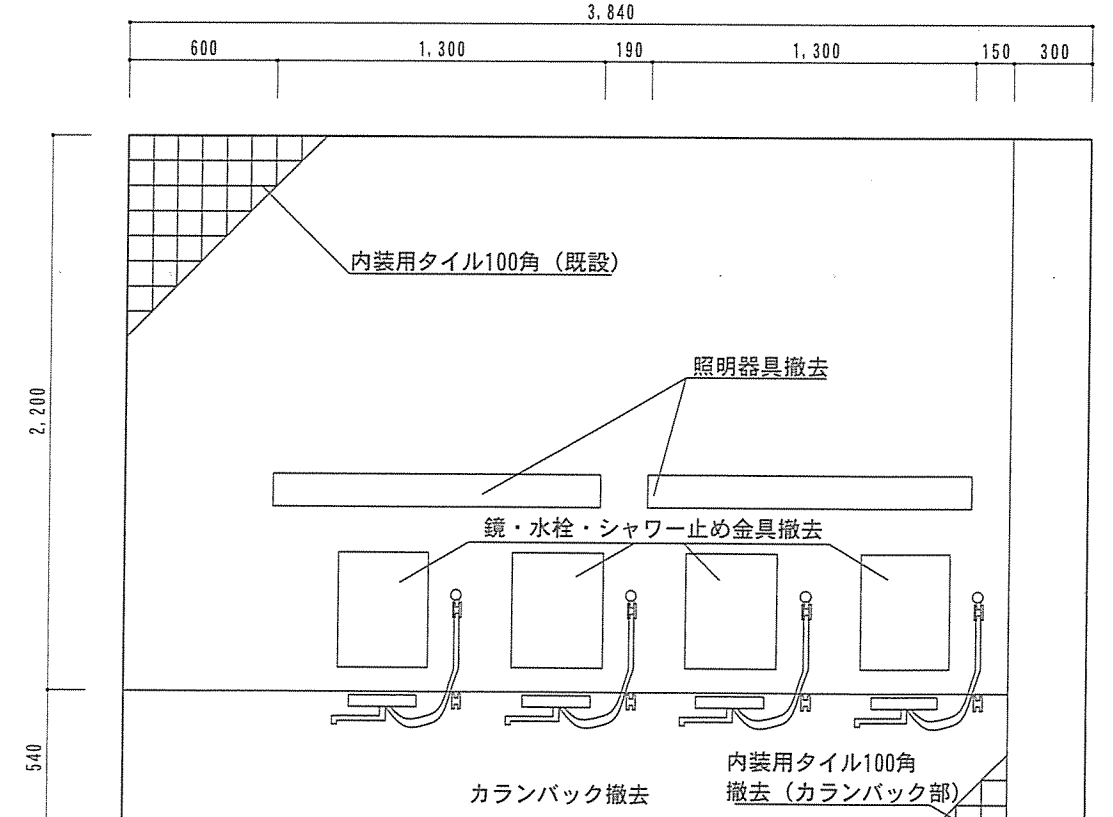
D面展開図 S=1/30 (整備前)
