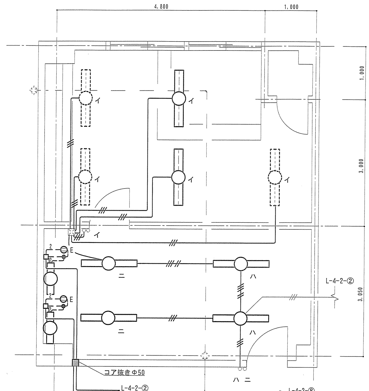
浴室・脱衣所電灯設備図 S=1/50
