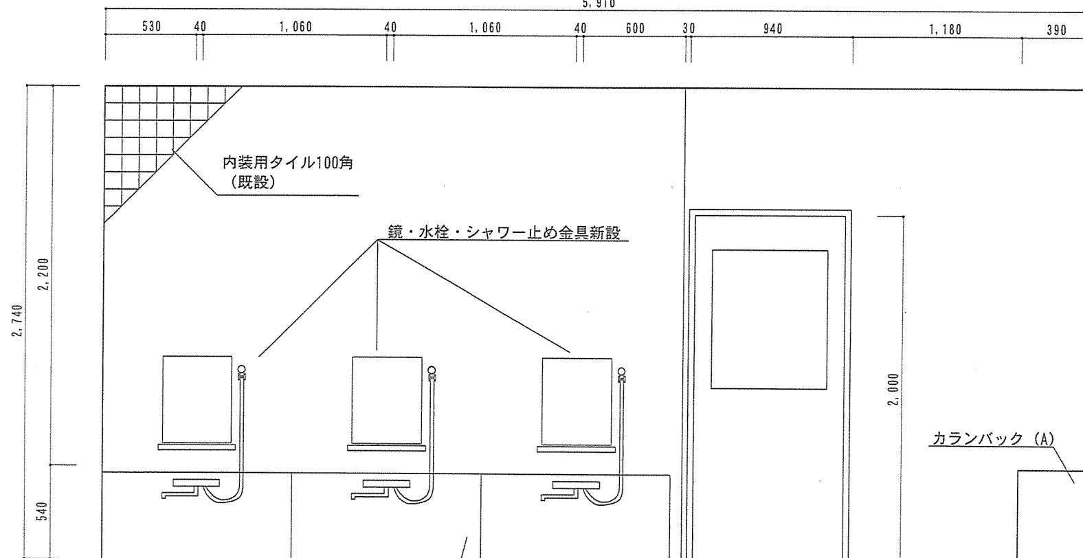
C面展開図 S=1/30 (整備後)
