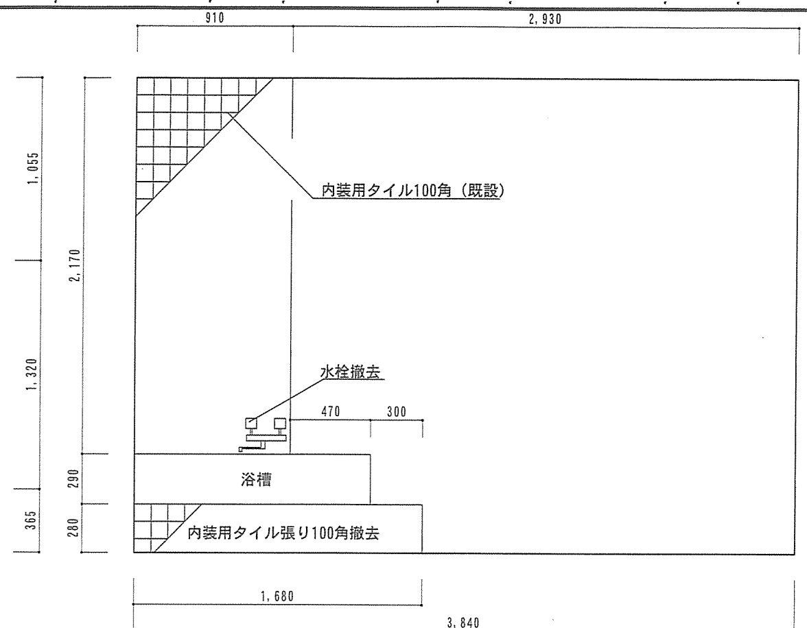
B面展開図 S=1/30 (整備前)
