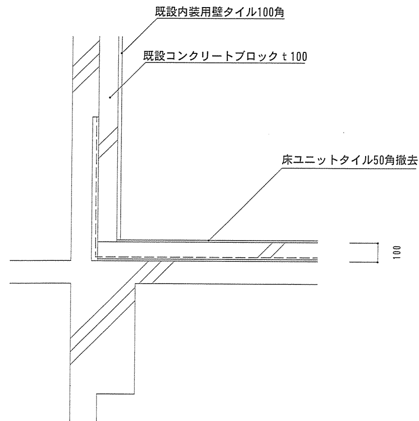
カラバック（B）・排水溝詳細図(整備前) S=1/20
