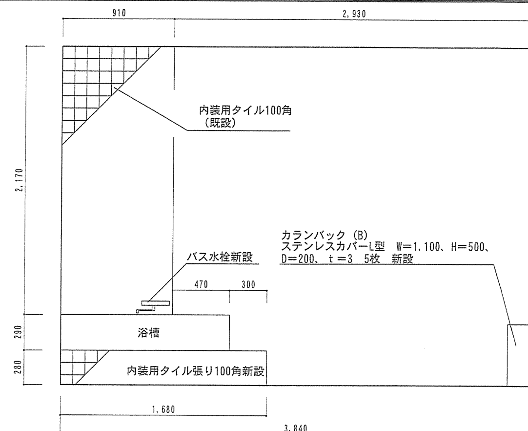
B面展開図 S=1/30 (整備後)
