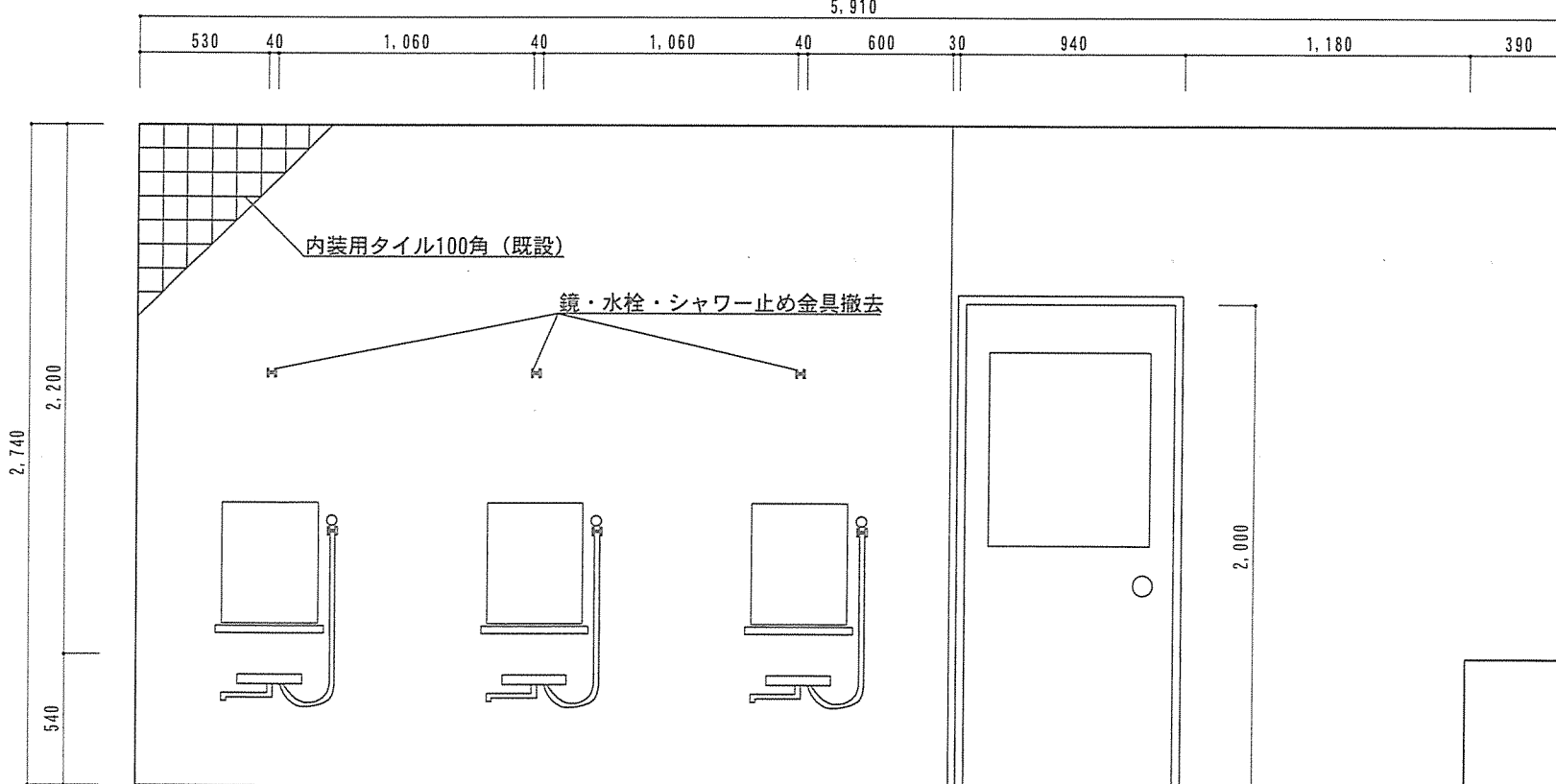
C面展開図 S=1/30 (整備前)
