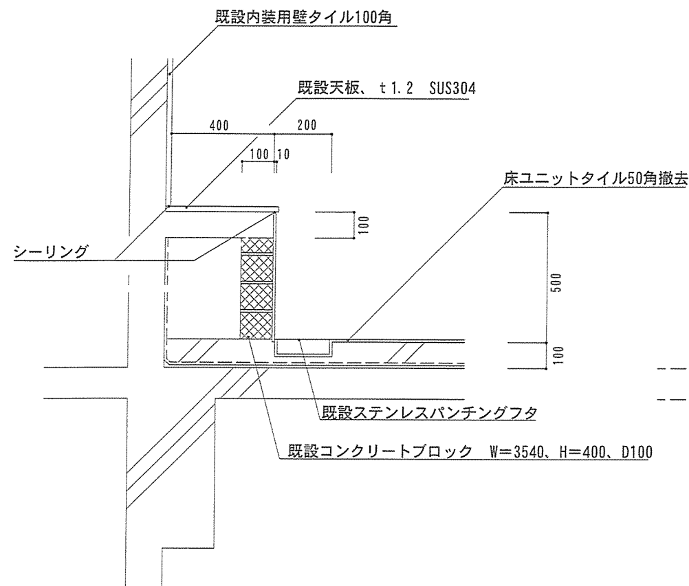
カラバック（A）・排水溝詳細図(整備前) S=1/20
