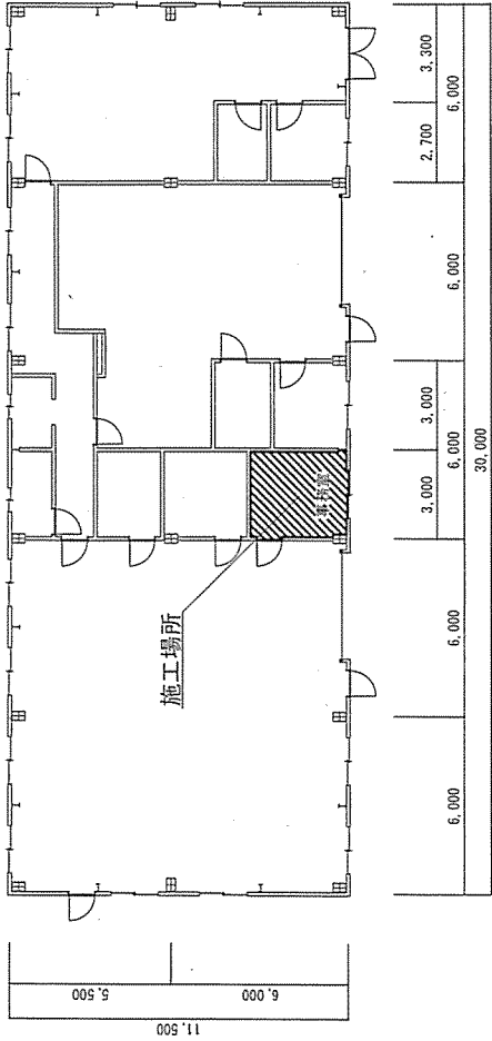
平面図 S = 1 : 200
