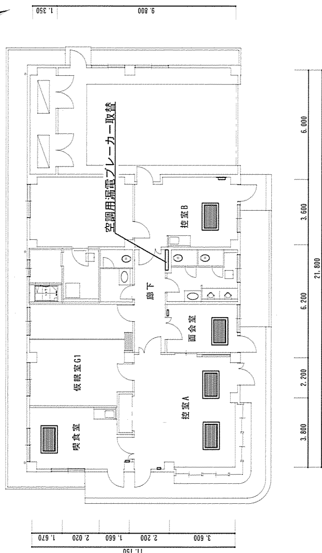
110号建物平面図 1/150
