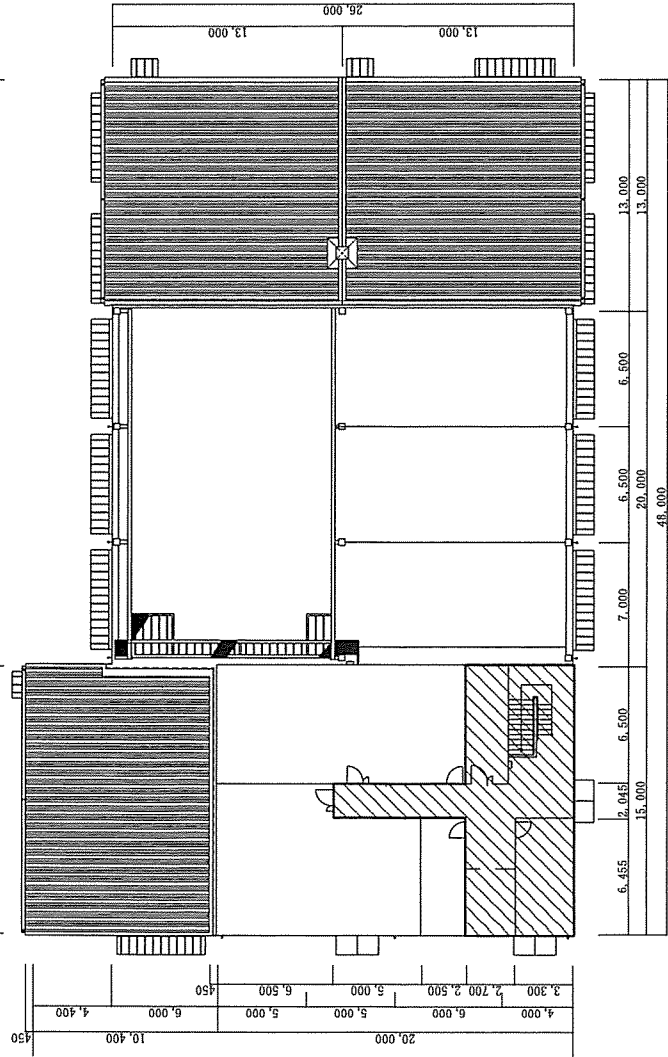
175号建物 2階平面図 S=1/300
