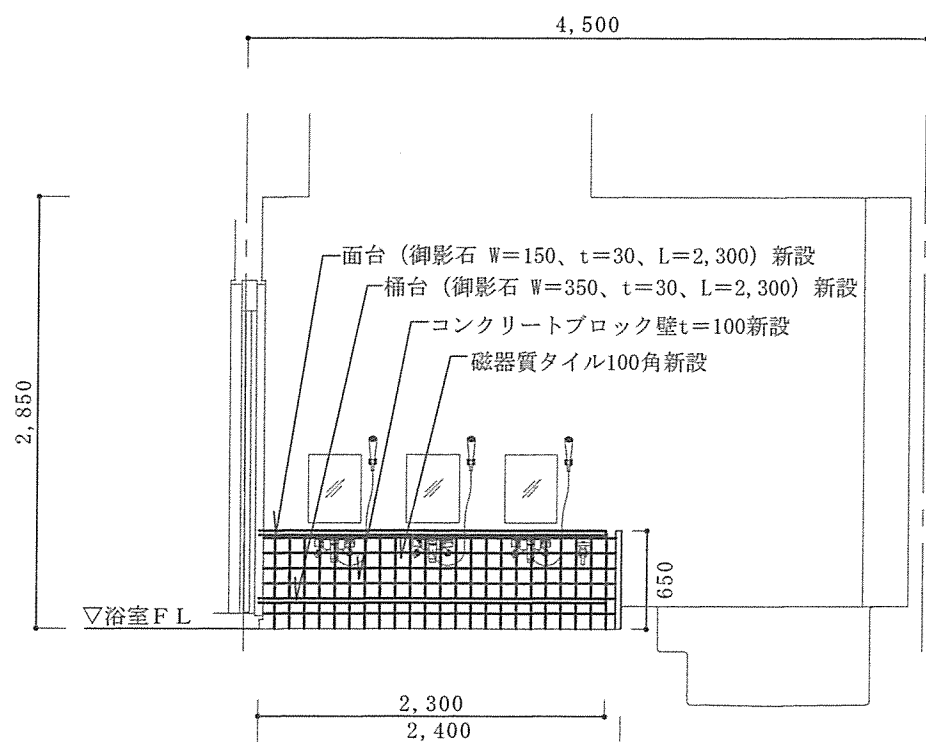
浴場展開図C面改修後 S=1/50
