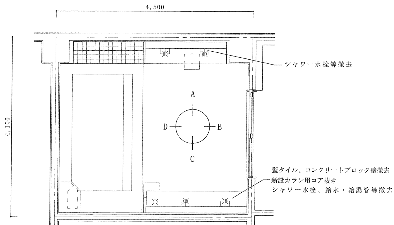
浴場平面図改修前 S=1/50
