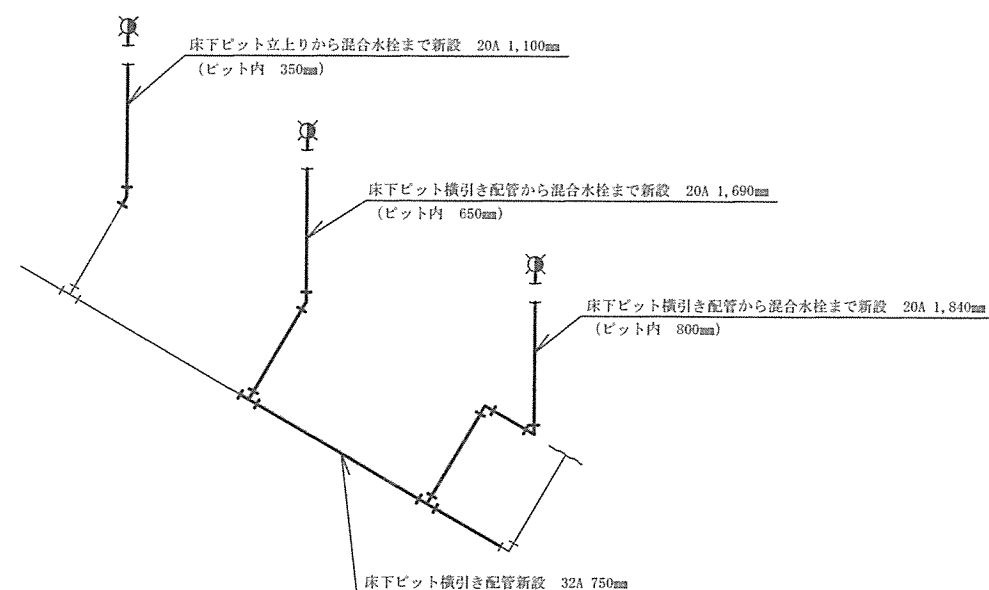
給湯管改修後 S=1/20
