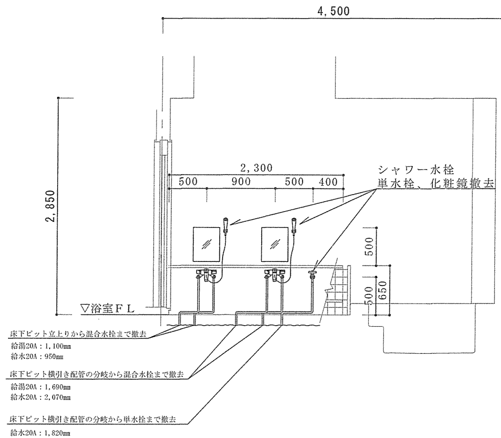
浴場展開図C面改修前 S=1/50
