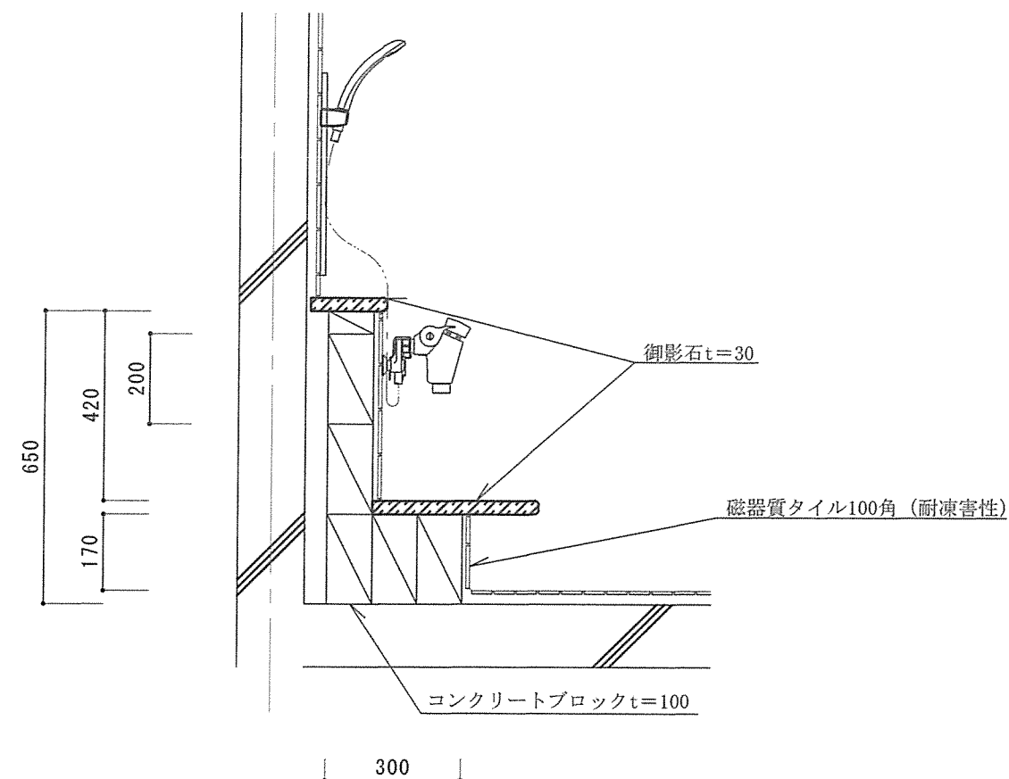
浴場カランバック詳細図 S=1/15
