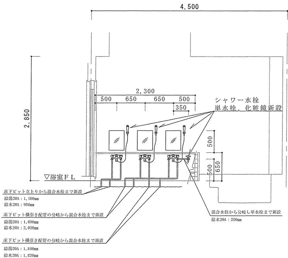
浴場展開図C面改修後 S=1/50
