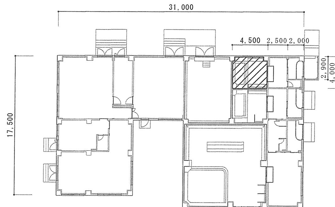
浴場平面図改修前 S=1/300
