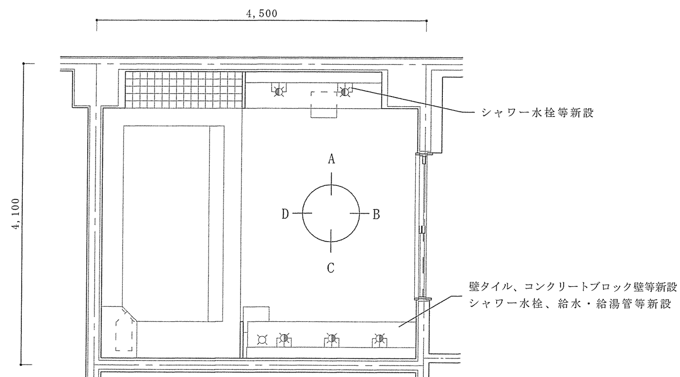
浴場平面図改修後 S=1/50
