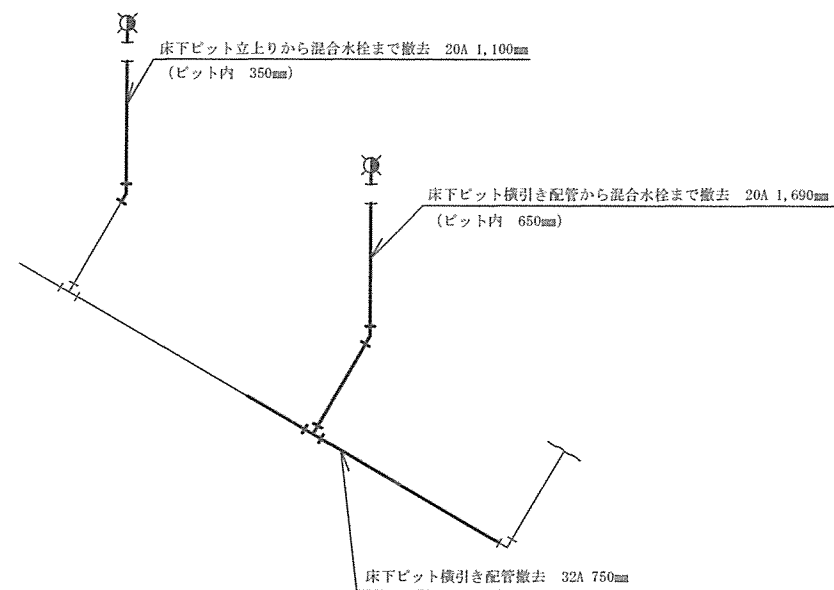
給湯管改修前 S=1/20
