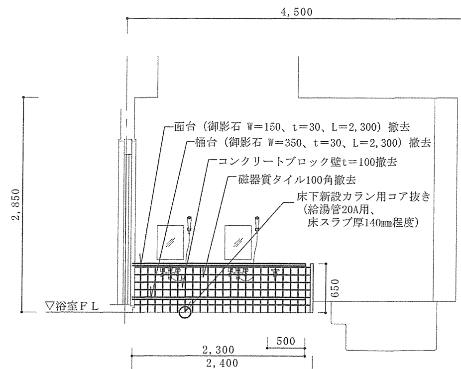
浴場展開図C面改修前 S=1/50
