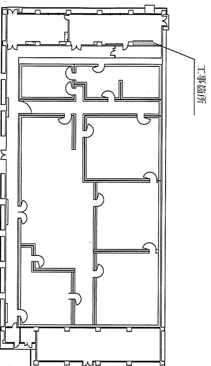
13号建物平面図 S=1/X
