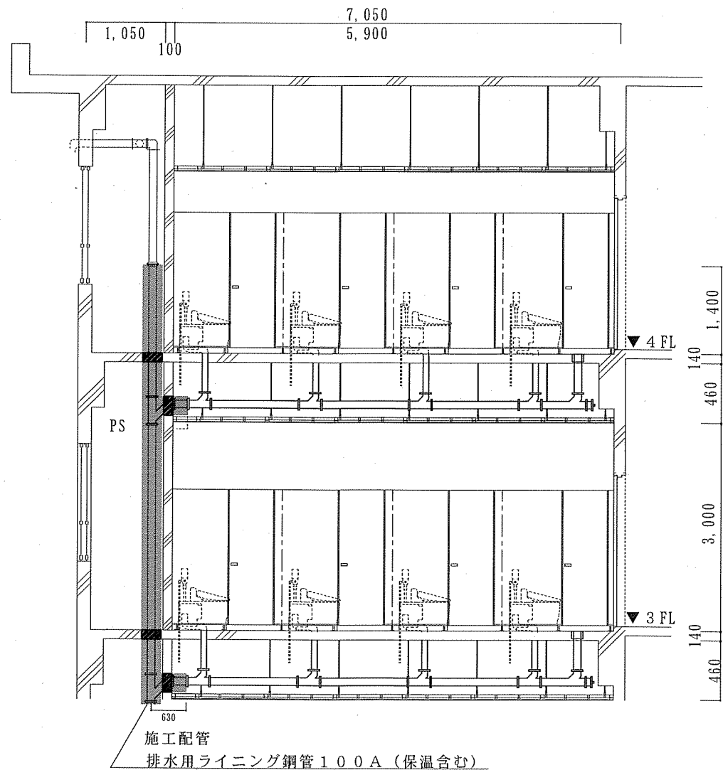
隊舎便所断面図 S = 1 / X
