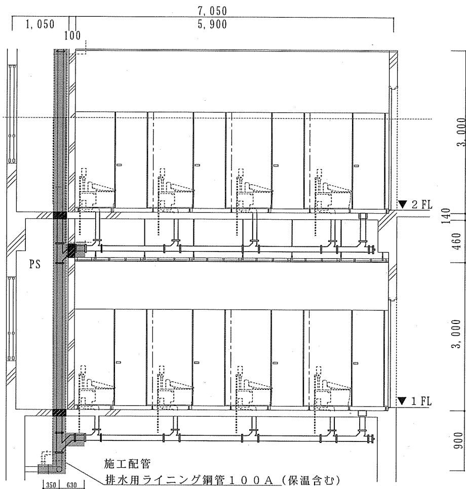
隊舎便所断面図 S = 1 / X
