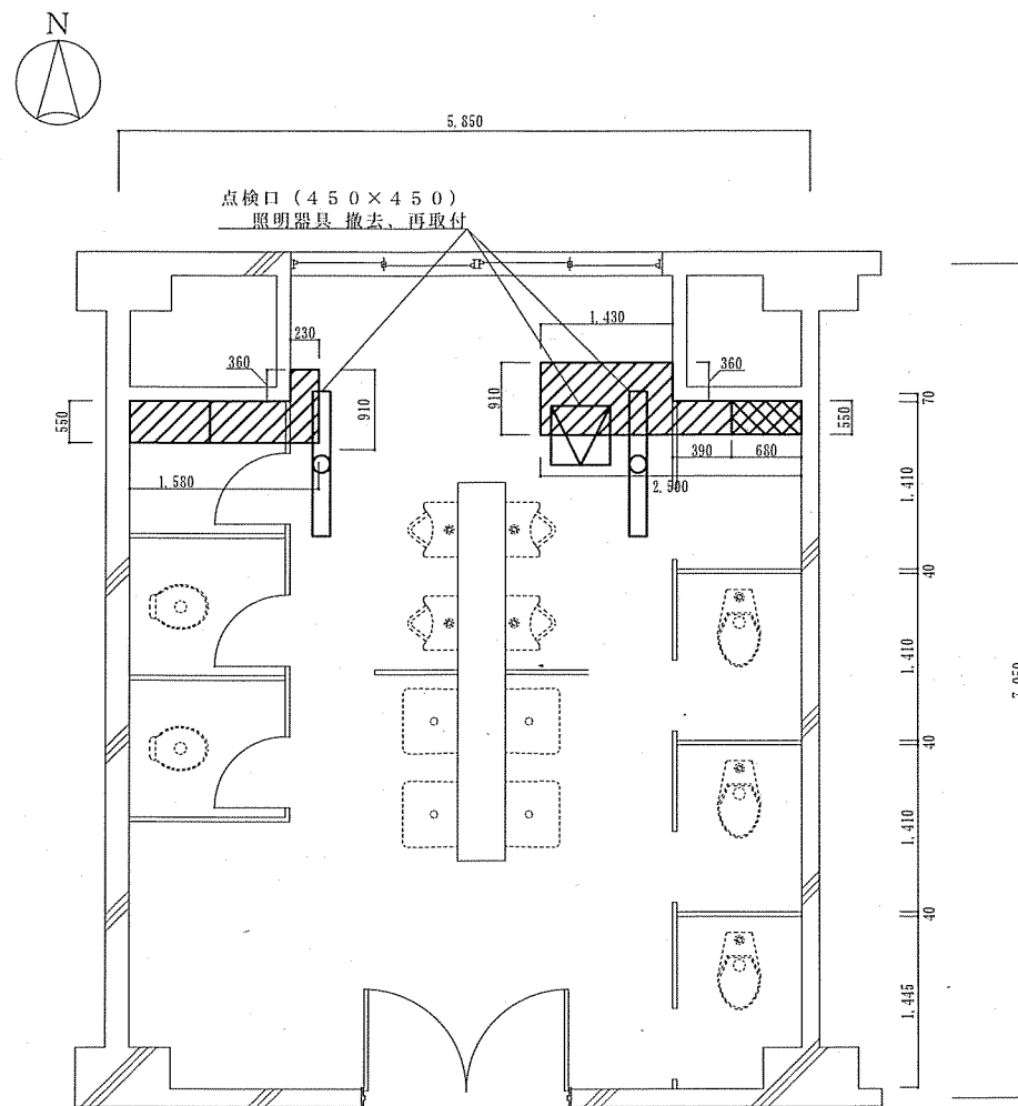
1F~3F 便所施工図 S = 1 / X
