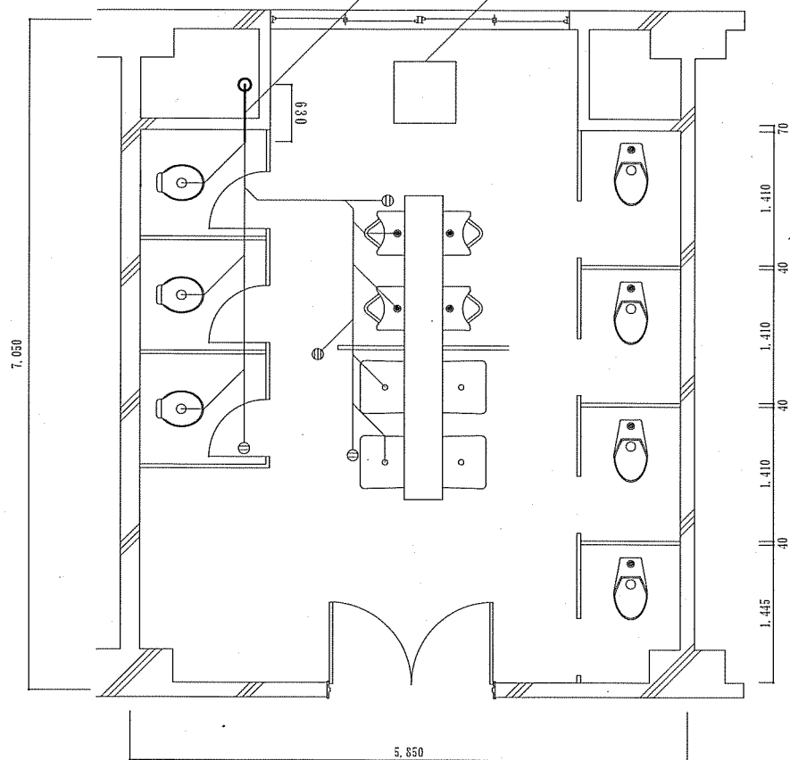
1F～4F 便所平面図 S = 1 / X
