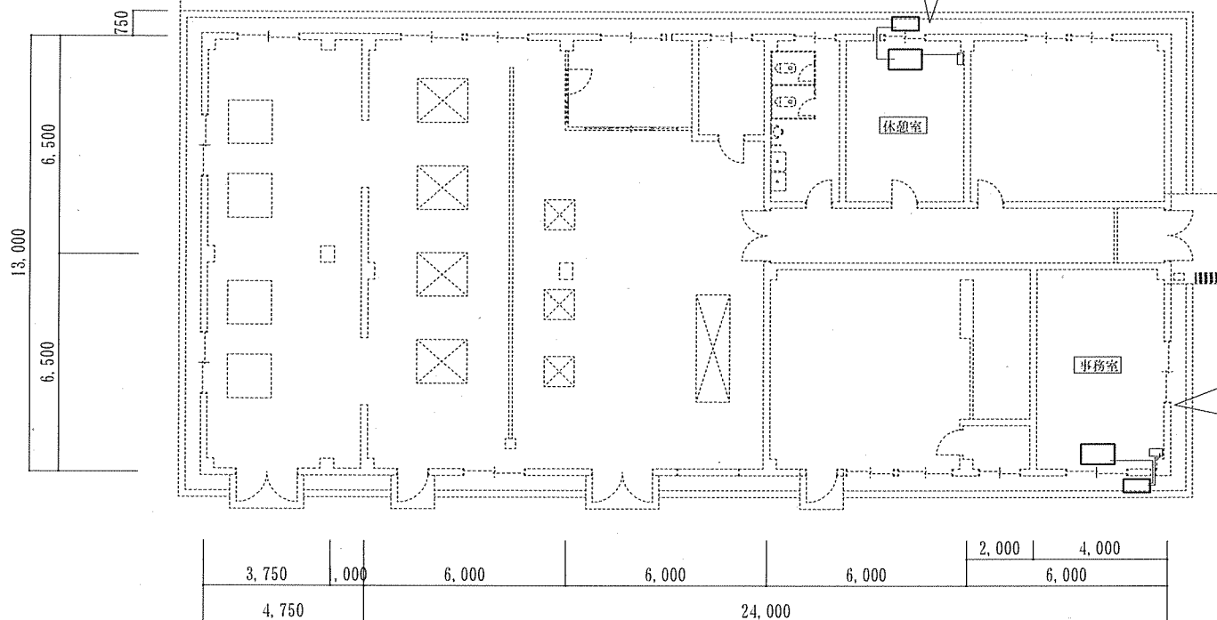
130号建物平面図 S=1/200
