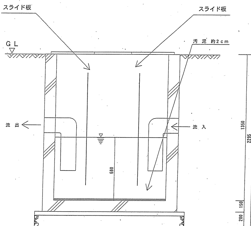
A-A断面図
