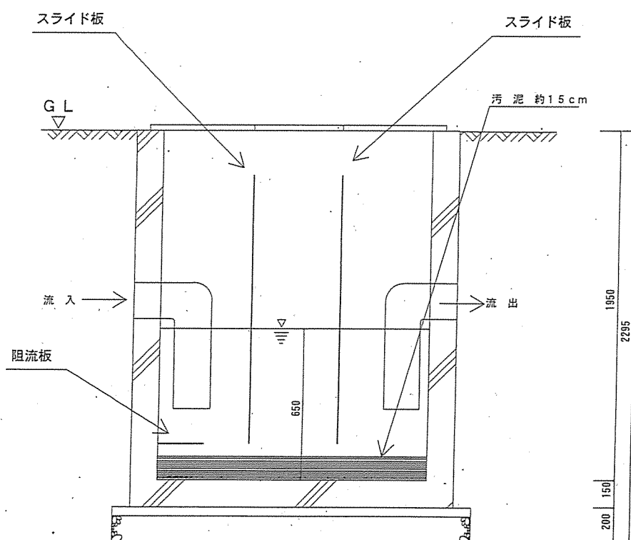
A-A断面図
