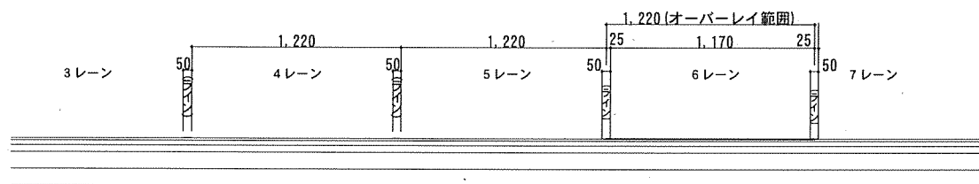
標準断面図 (A-A') 1:600
