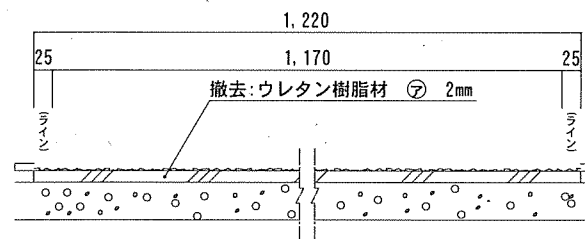
施工前標準断面図 NO SCALE
