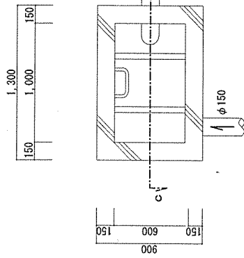
油分離槽③-平面図 1:30
