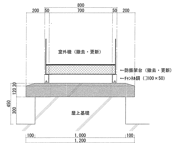
屋上機械基礎廻り詳細図 S=1/20
