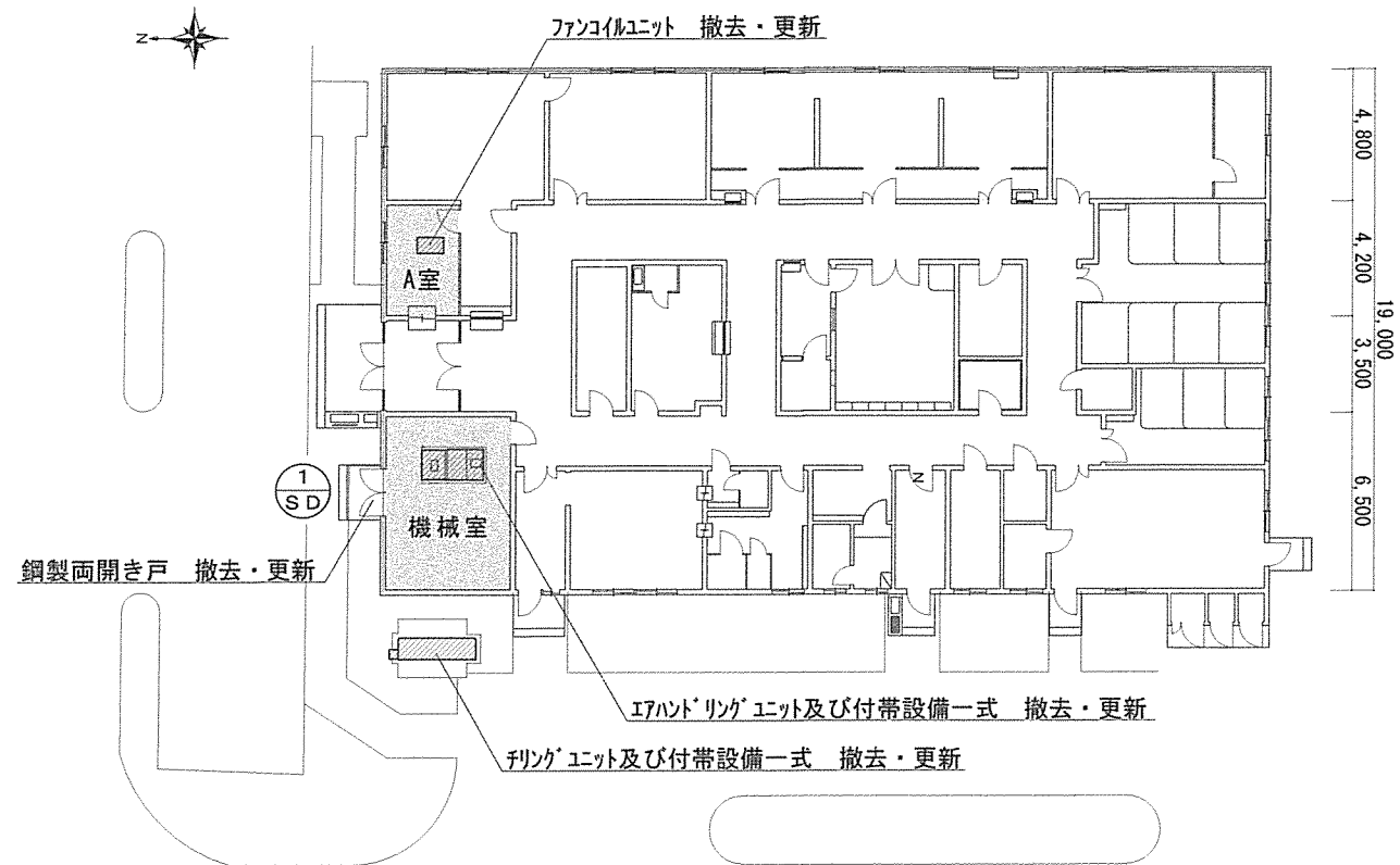
131号建物配置平面図 S=1/300
