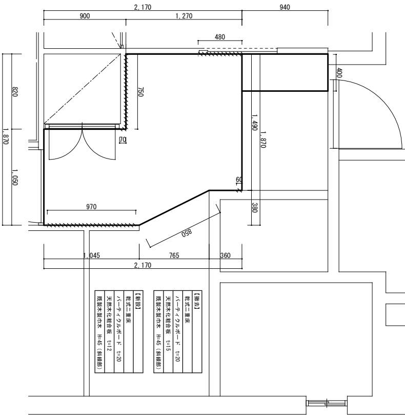
標準詳細平面図 S=1:40
