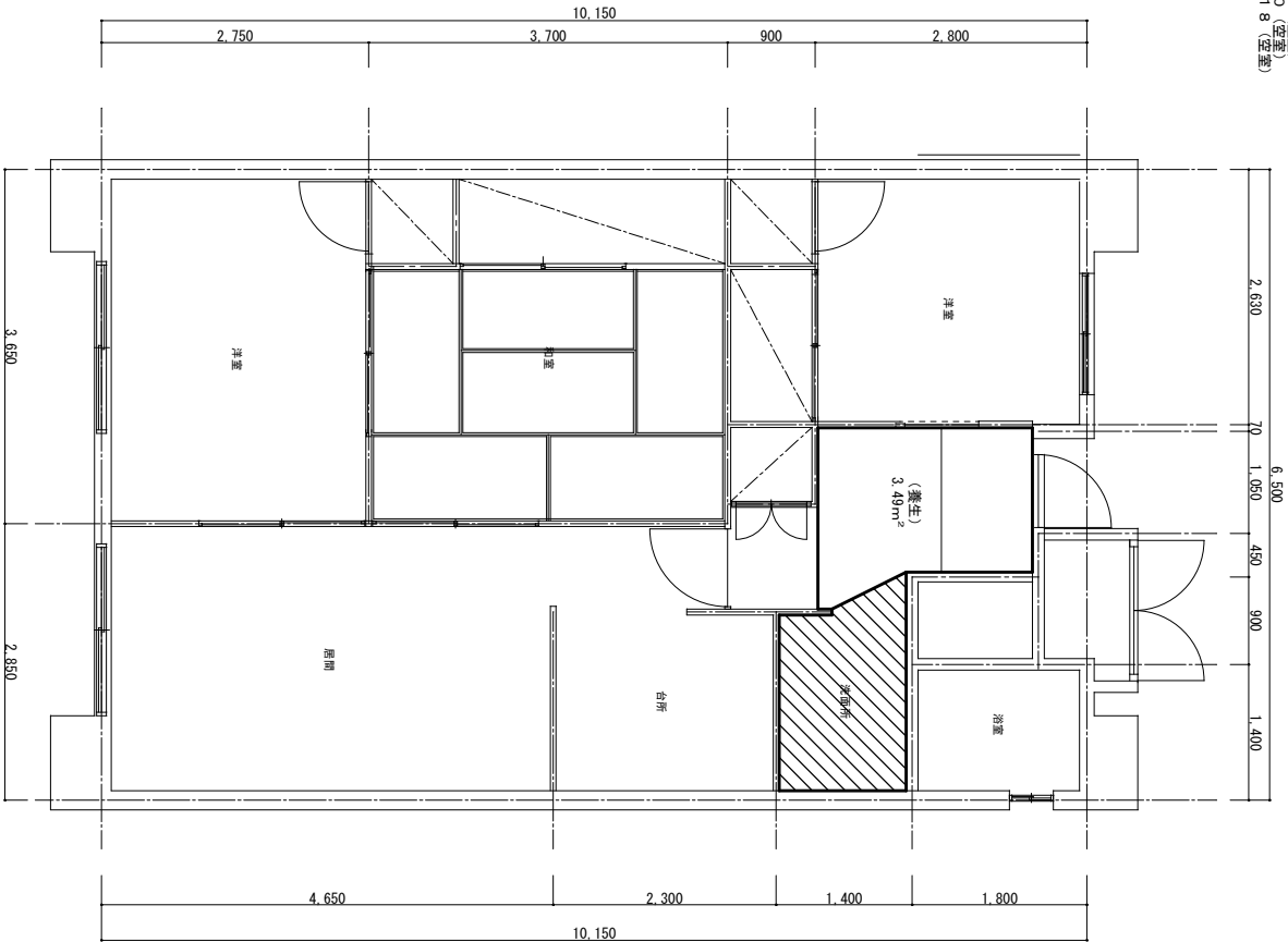
標準平面図 S-1:60
