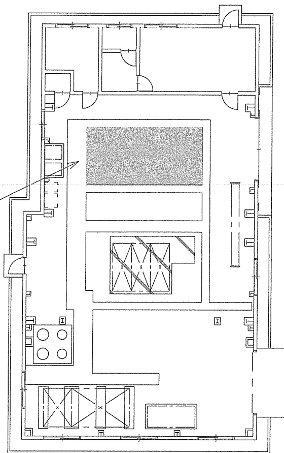
ボイラー室平面図 S=1/Non
