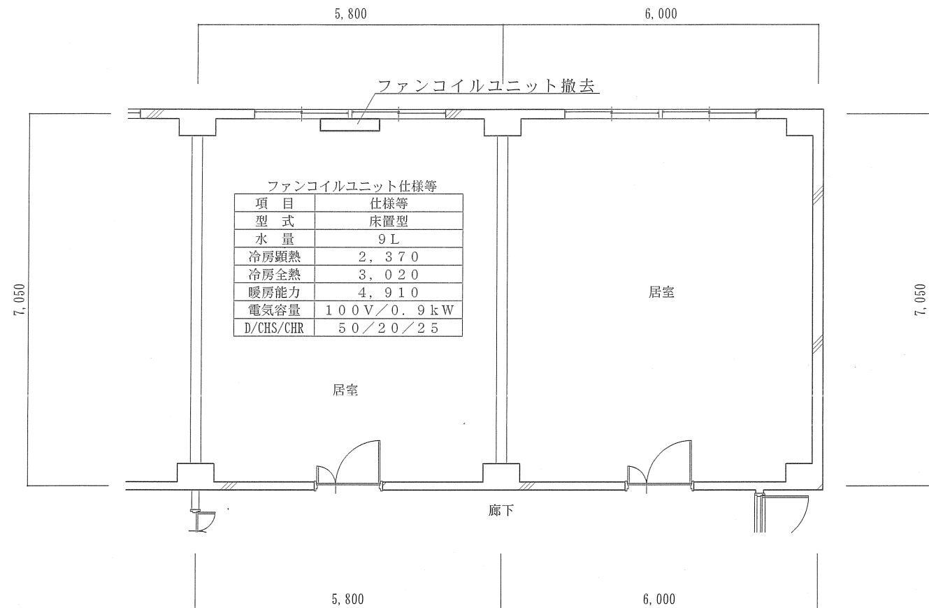
3階居室改修前平面図 S=1:100
