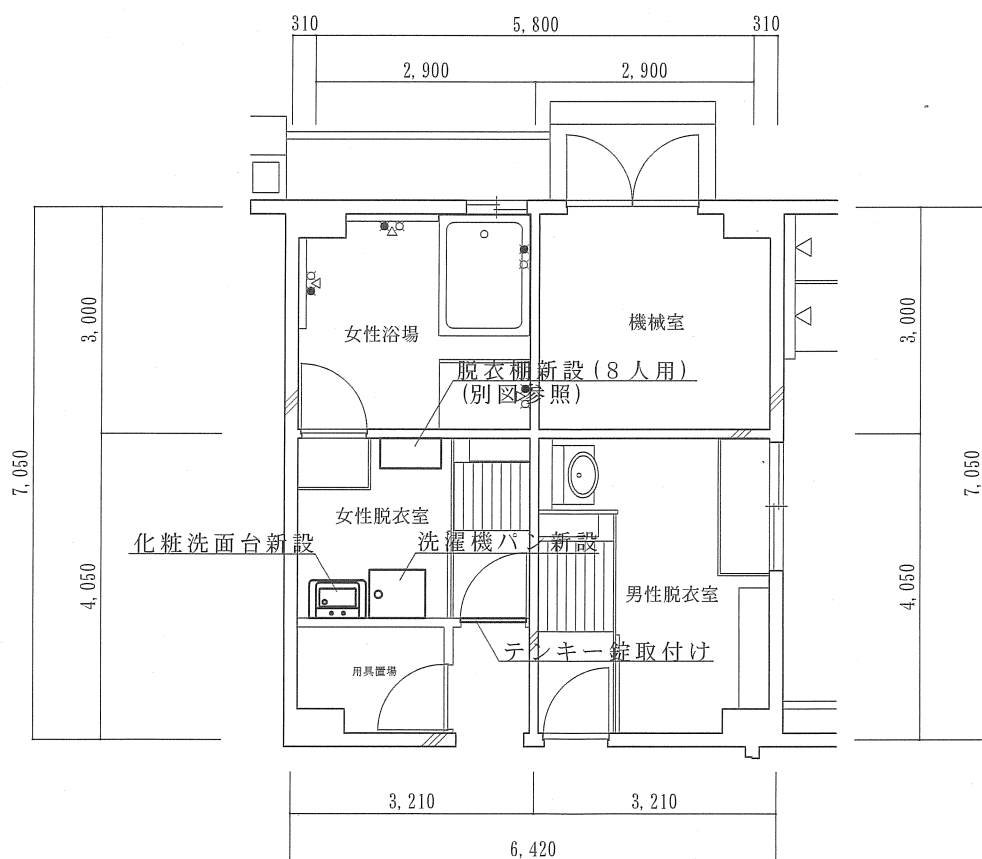
1階女性脱衣室改修後平面図 S=1:100
