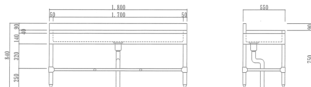
既設ステンレス製洗面流し台正面・側面図 S=1:20
