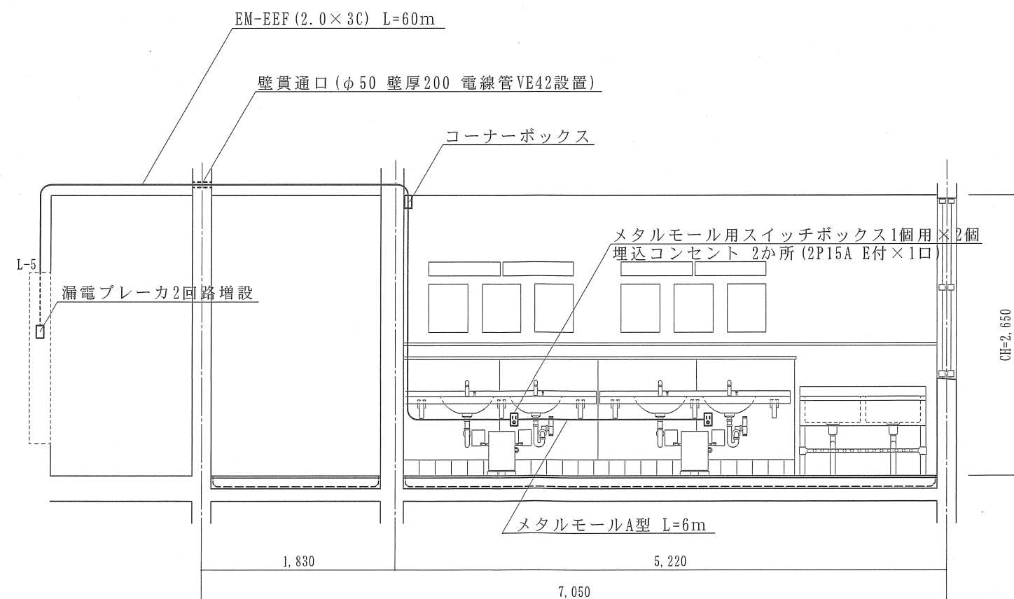
3階女性用洗面・洗濯室新設電気配線図 S=1:50
