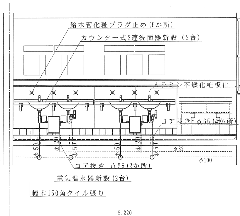
3 階女性用洗面・洗濯室改修後正面図 S=1:50
