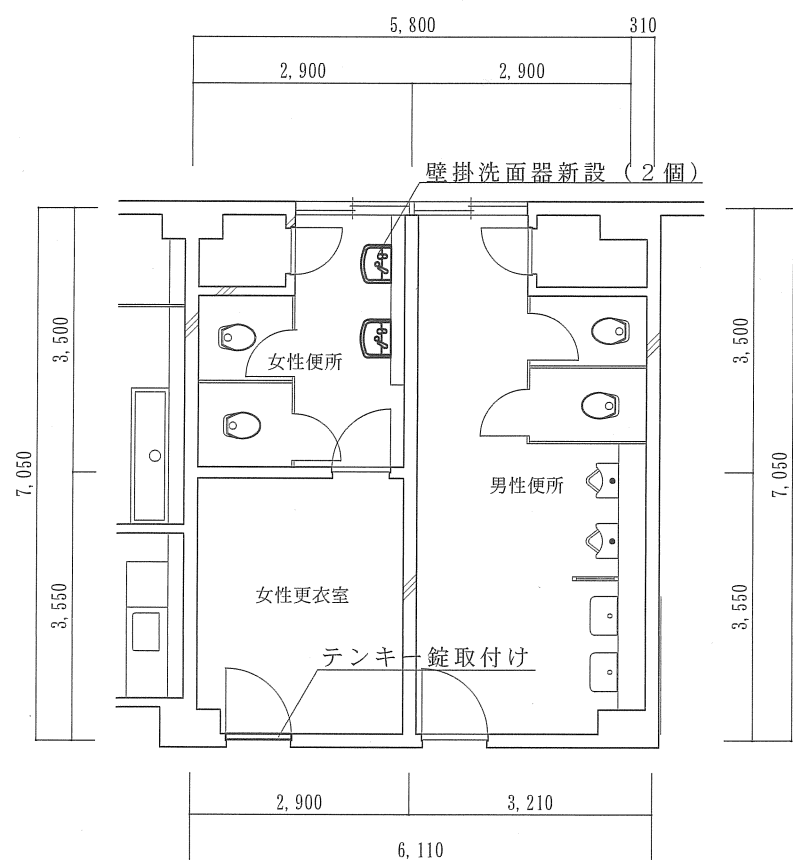
2階女性便所改修後平面図 S=1:100
