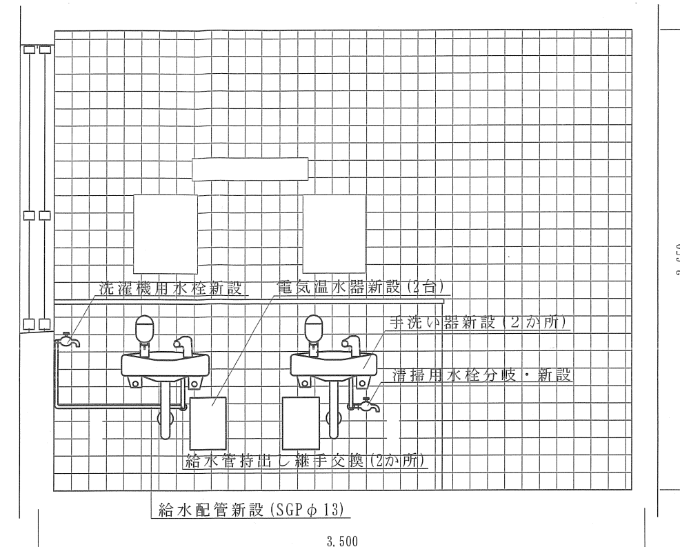
2階女性便所改修後断面図 S=1:30
