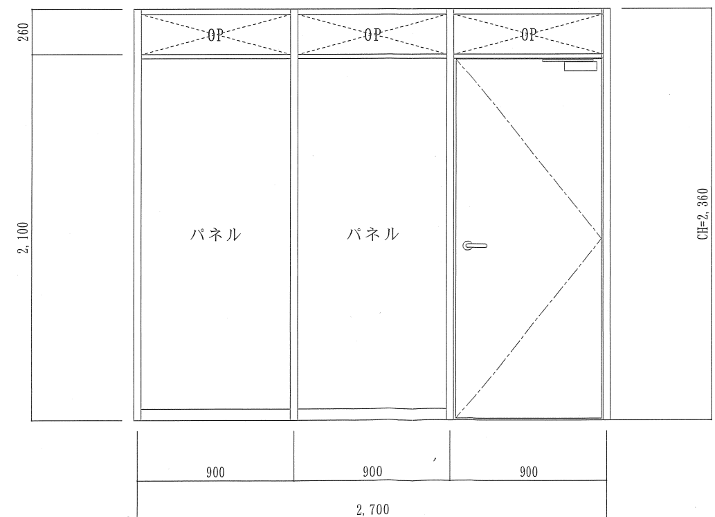
アルミパーテーション短辺正面図 S=1:30
