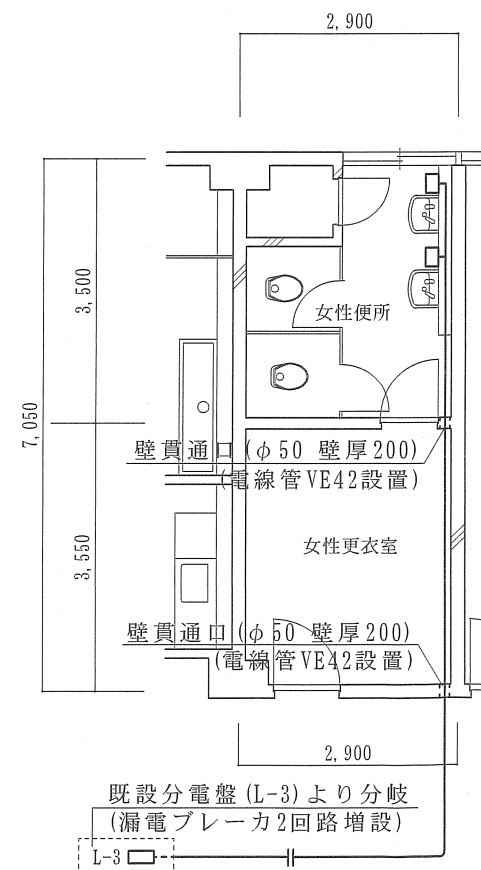
2階女性便所新設電気配線図 S=1:30
