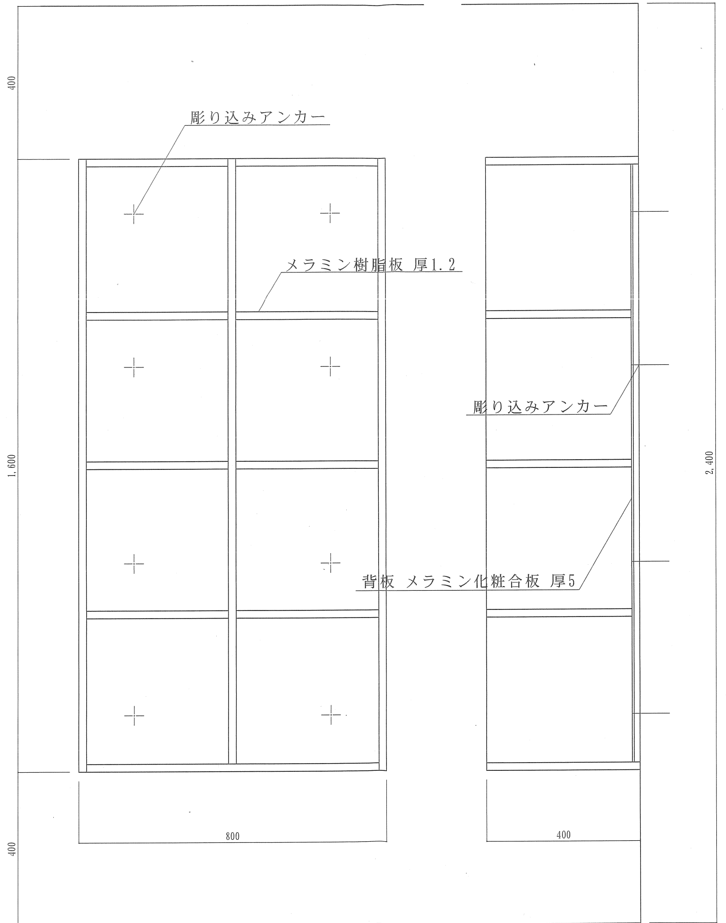
脱衣棚 (新設) S=1:10
