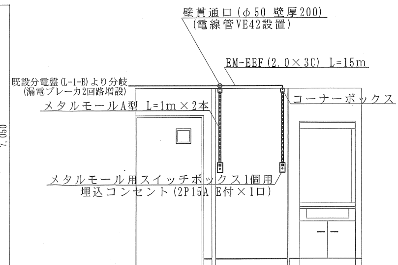
1階女性脱衣室新設電気配線図 S=1:100
