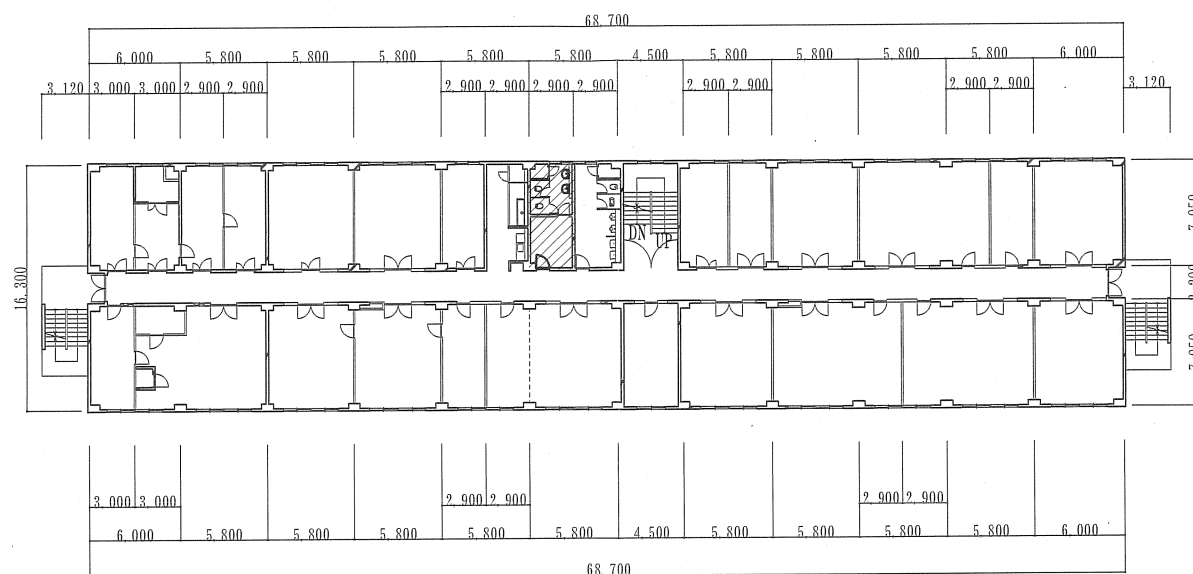
2 階改修後平面図 S=1:500
