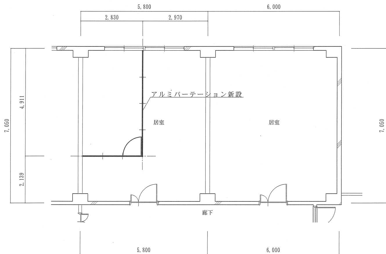
3階居室改修後平面図 S=1:100
