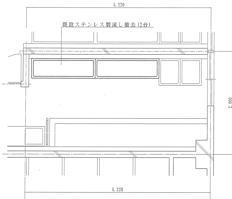
3 階女性用洗面・洗濯室改修前平面図 S=1:50
