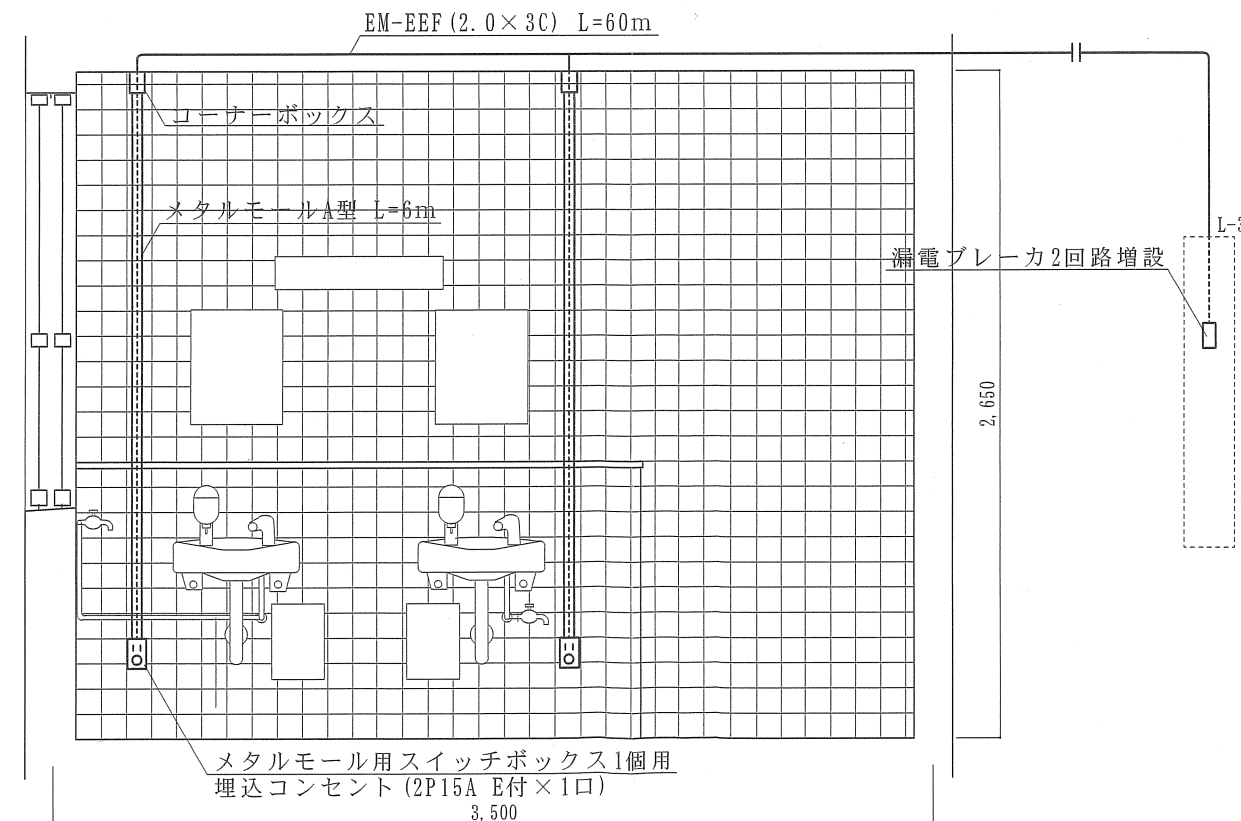
2階女性便所新設電気配線図 S=1:30
