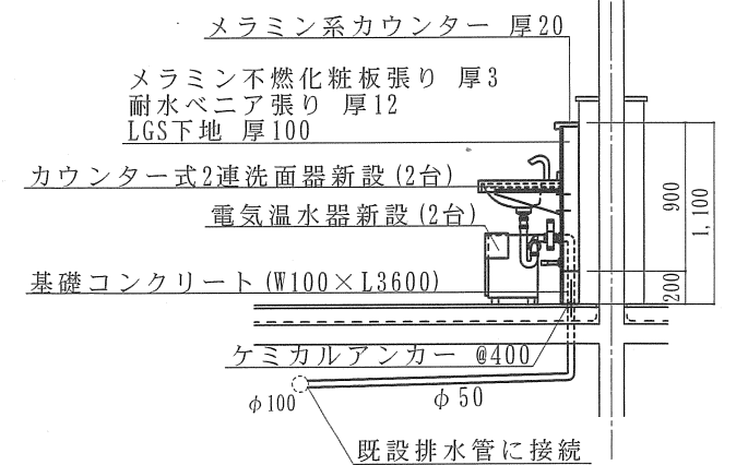
3 階女性用洗面・洗濯室断面図 S=1:50
