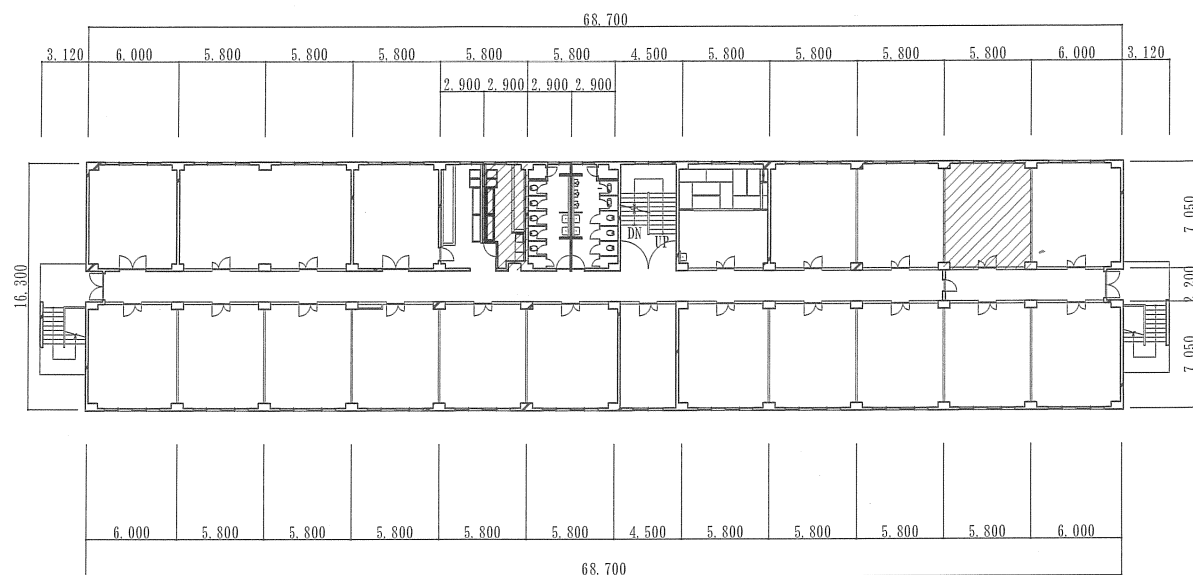
3 階改修前平面図 S=1:500
