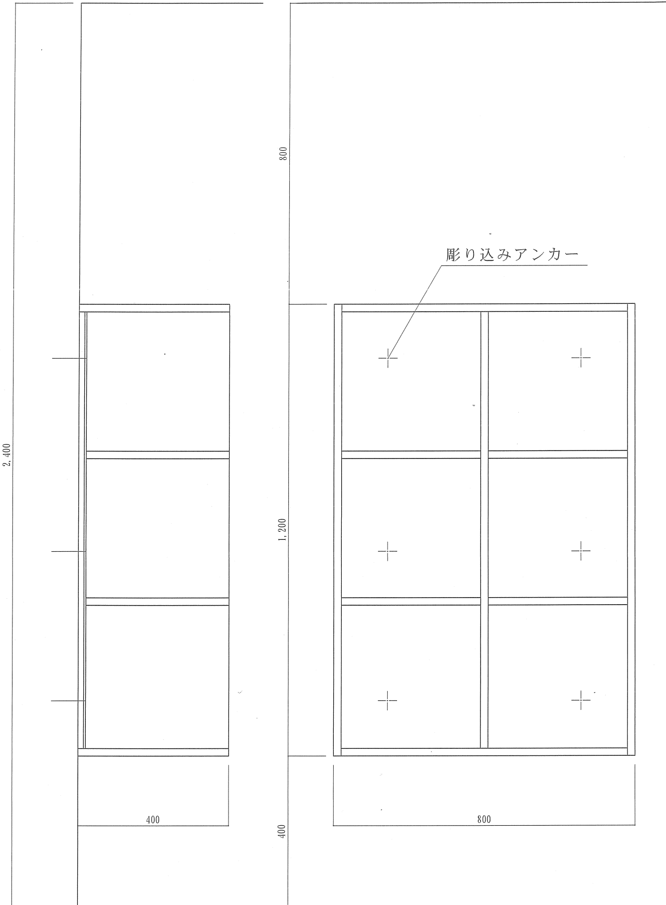
既設脱衣棚 (撤去) S=1:10
