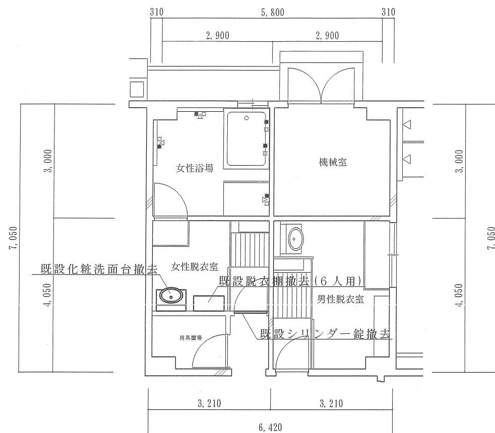
1階女性脱衣室改修前平面図 S=1:100
