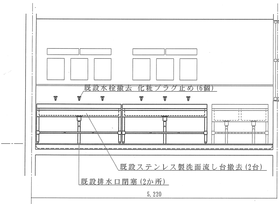
3 階女性用洗面・洗濯室改修前正面図 S=1:50
