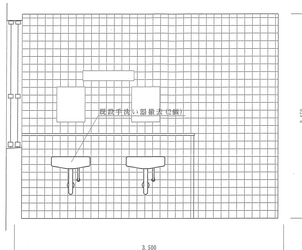
2階女性便所改修前断面図 S=1:30
