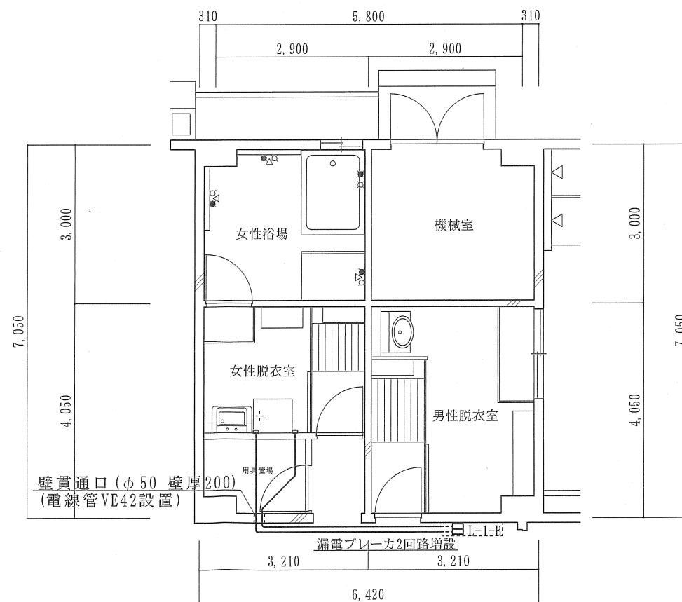
1階女性脱衣室新設電気配線図 S=1:100
