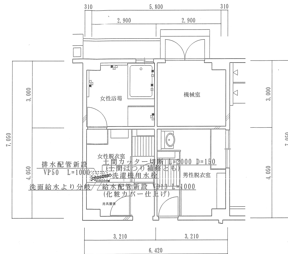
1階女性脱衣室給排水設備図 S=1:100
