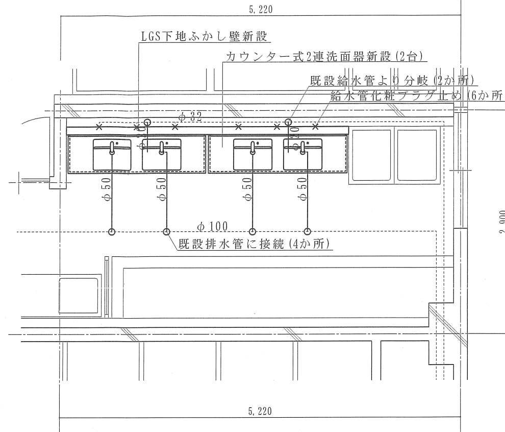
3 階女性用洗面・洗濯室改修後平面図 S=1:50
