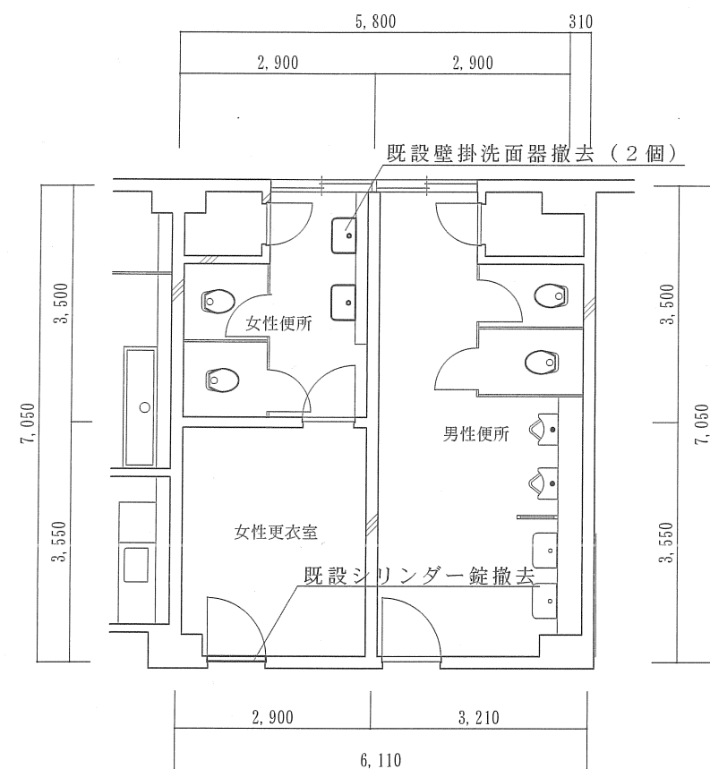
2階女性便所改修前平面図 S=1:100
