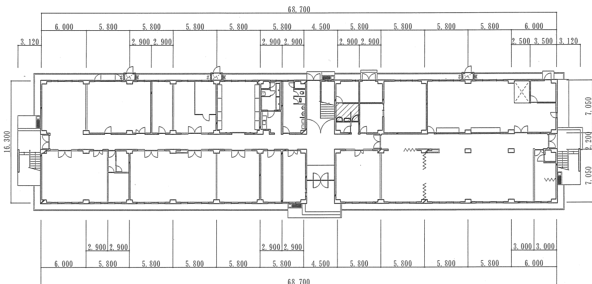
1 階改修前平面図 S=1:500
