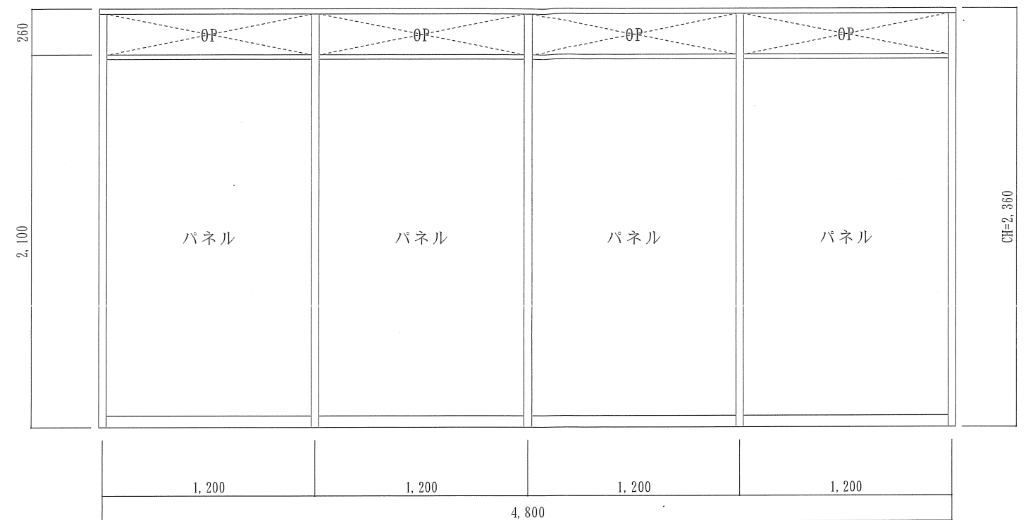
アルミパーテーション長辺正面図 S=1:30
