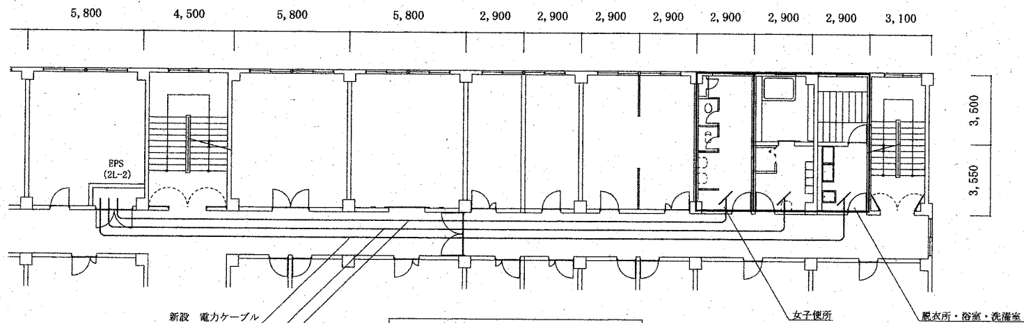
3号建物2階平面図（電気設備）
