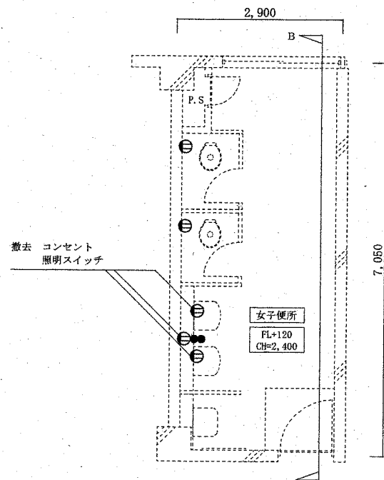
女子便所 (改修前) 平面図 (コンセント)
