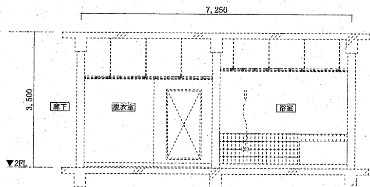
D部 断面詳細図
