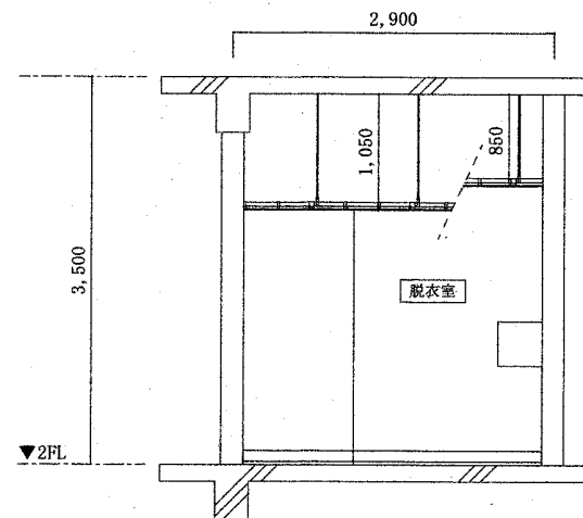
C部 断面詳細図
