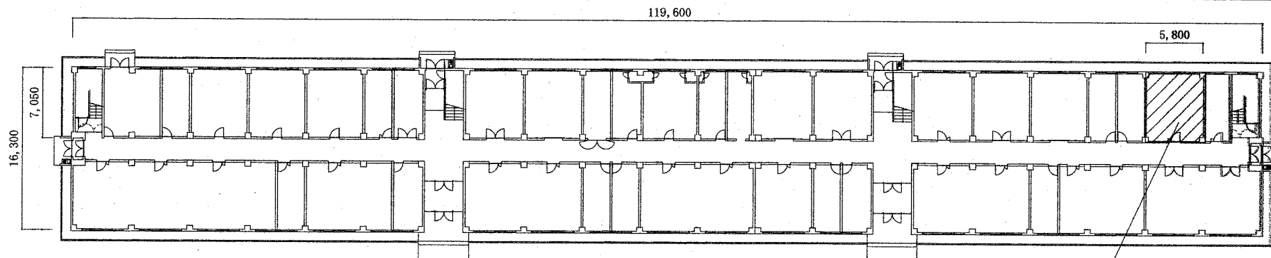
3号建物1階 平面図
