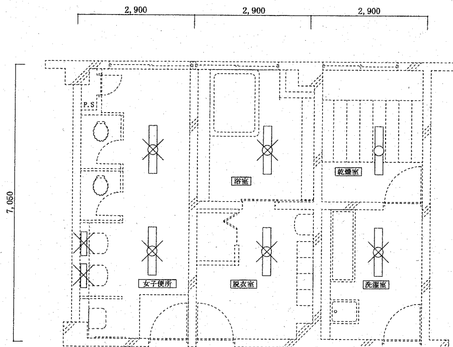
女子便所・脱衣所・浴室・洗濯室（改修前）平面図（照明設備）
