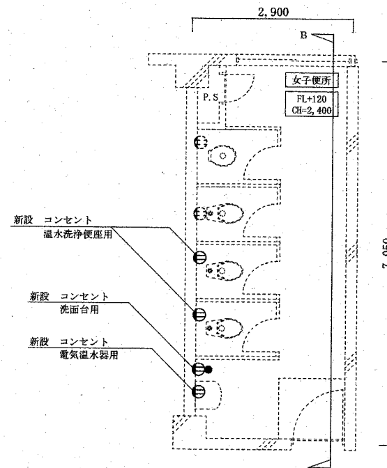
女子便所 (改修後) 平面図 (コンセント)
