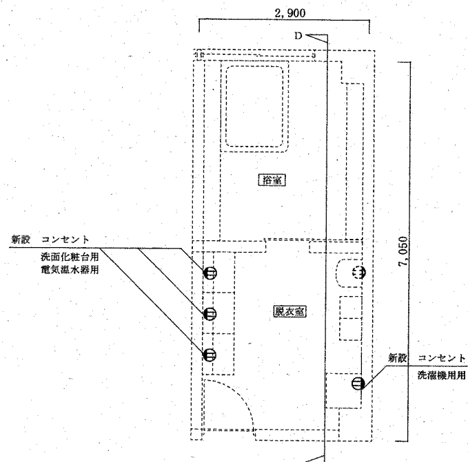
脱衣所・浴室（改修後）平面図（コンセント）
