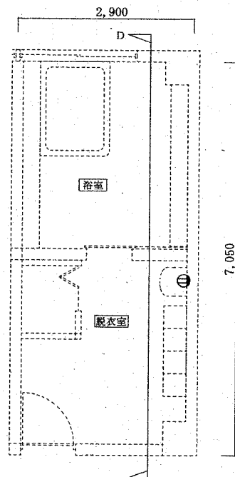
脱衣所・浴室（改修前）平面図（コンセント）
