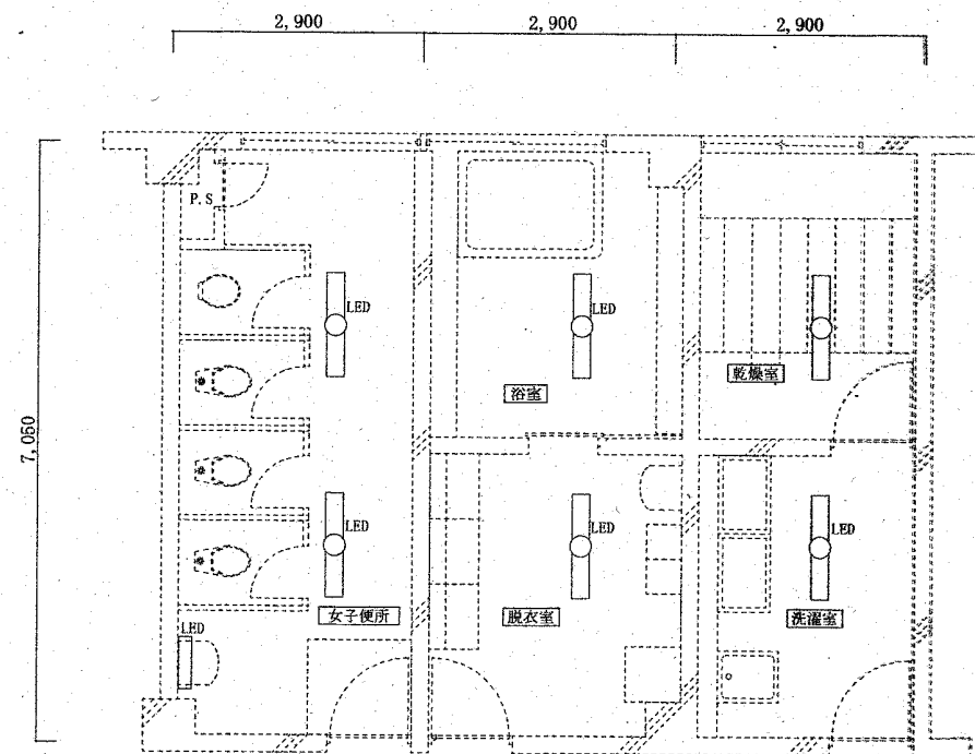
女子便所・脱衣所・浴室・洗濯室（改修後）平面図（照明設備）
