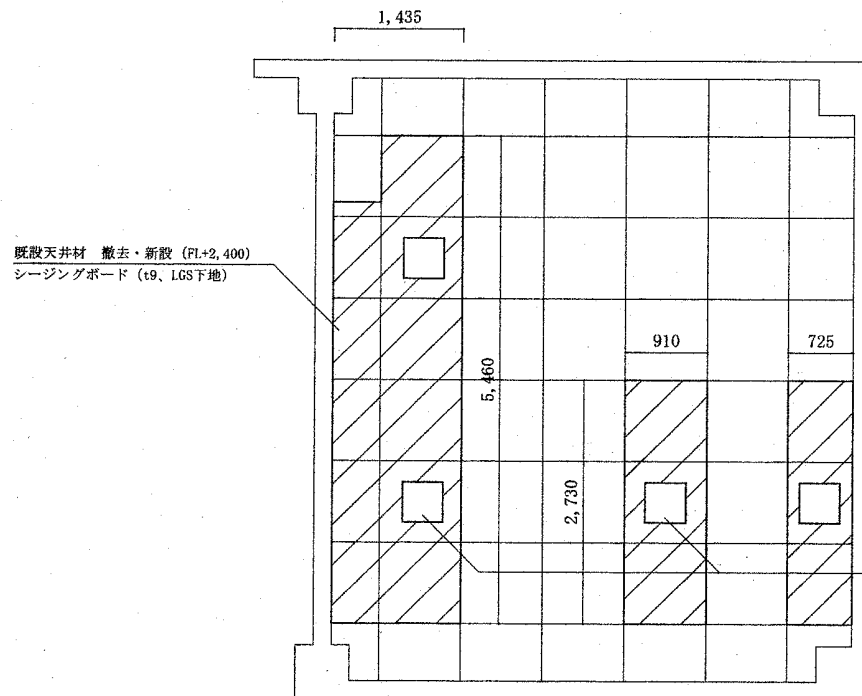
更衣室 天井伏図 (施工前・後)
