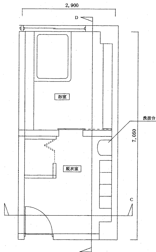
脱衣所・浴室（改修前）平面図
