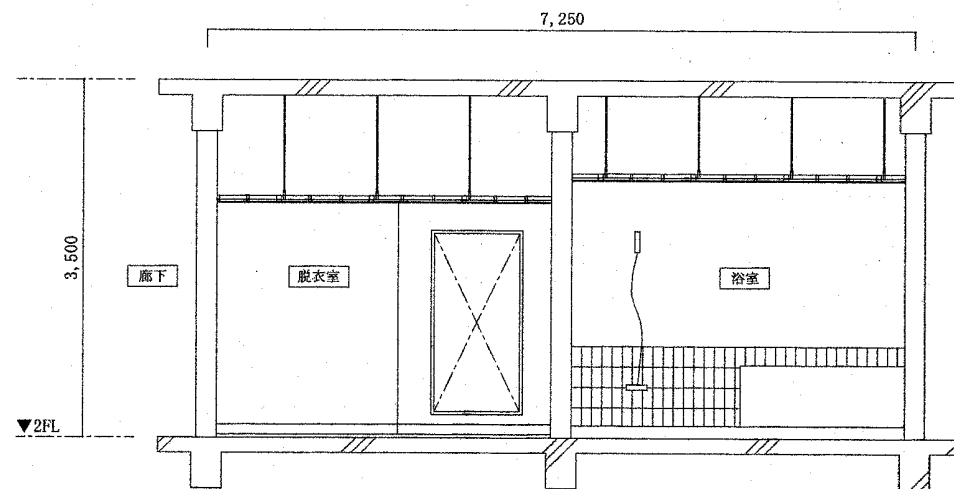
D部 断面詳細図
