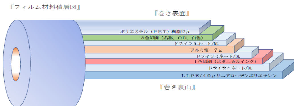
図1—材料・構造（断面図）
