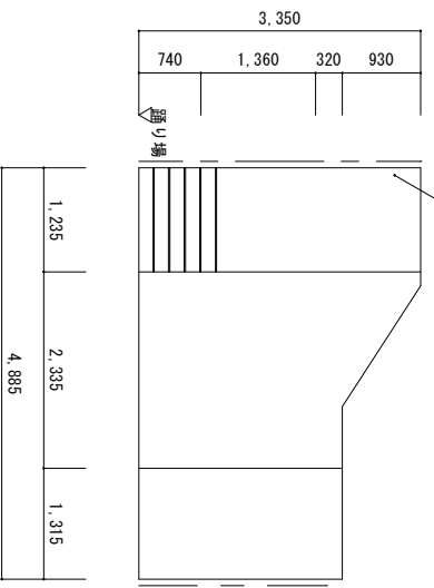
【改修前】工事箇所-B-展開図 (A) 1 : 100
