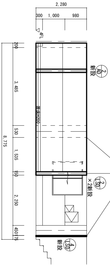
【改修後】工事箇所-A- 展開図 (b) 1 : 100
