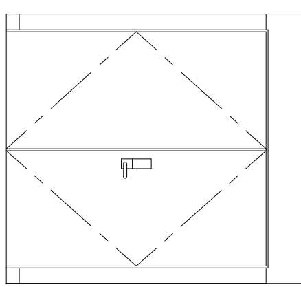
③SD × 1 軽量鋼製フラッシュ面開き扉
