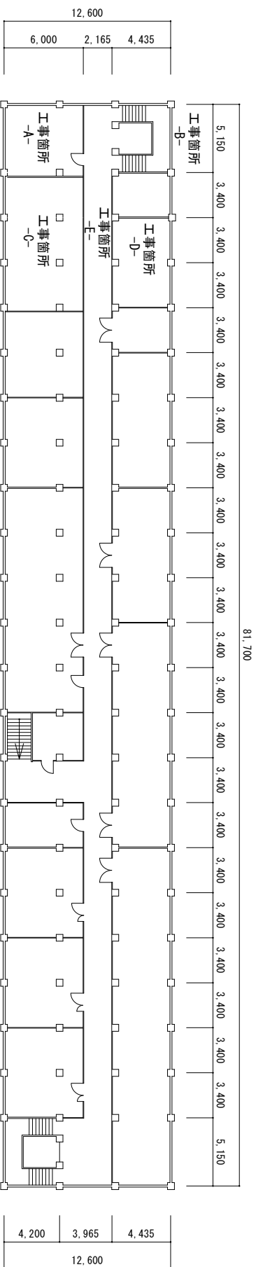
1号隊舎4階 平面図 1:400
