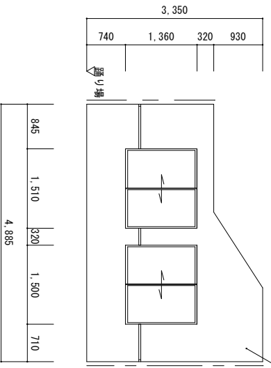
【改修前】工事箇所-B-展開図 (C) 1 : 100
