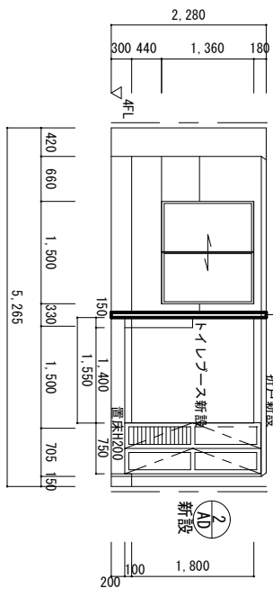
【改修後】工事箇所-A- 展開図 (a) 1 : 100
