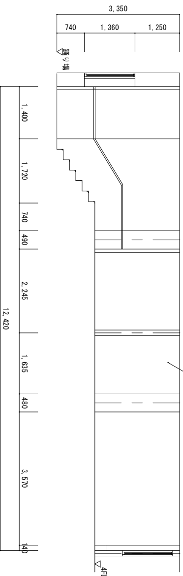
【改修前】工事箇所-A- 展開図 (d-D) 1 : 100
