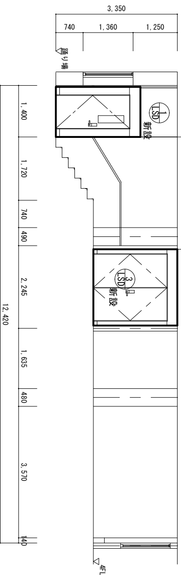
【改修後】工事箇所-A- 展開図 (d-D) 1 : 100
