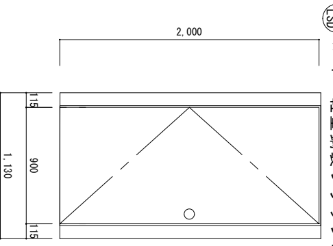
④SD × 1 軽量鋼製フラッシュ片開き扉
