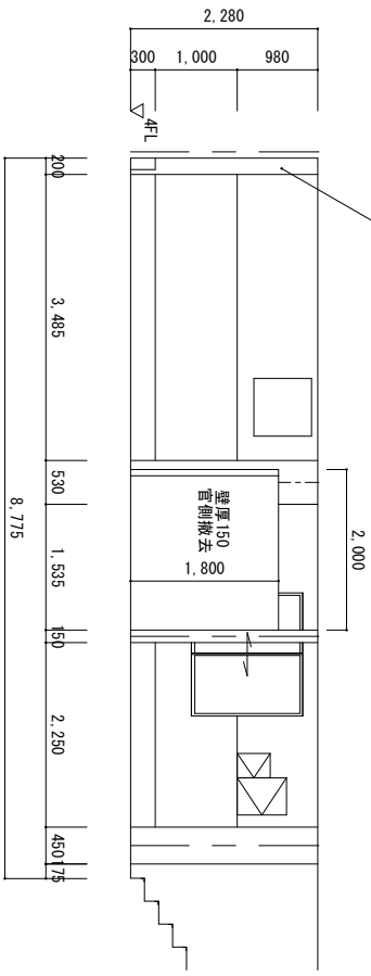
【改修前】工事箇所-A- 展開図 (b) 1 : 100
