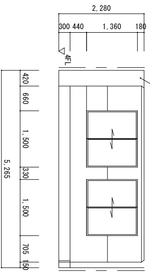
【改修前】工事箇所-A- 展開図 (a) 1 : 100
