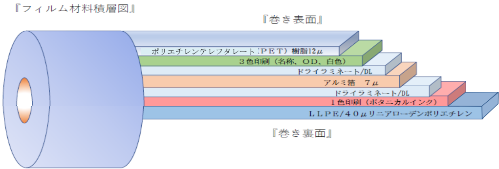
図1－材料・構造（断面図）
