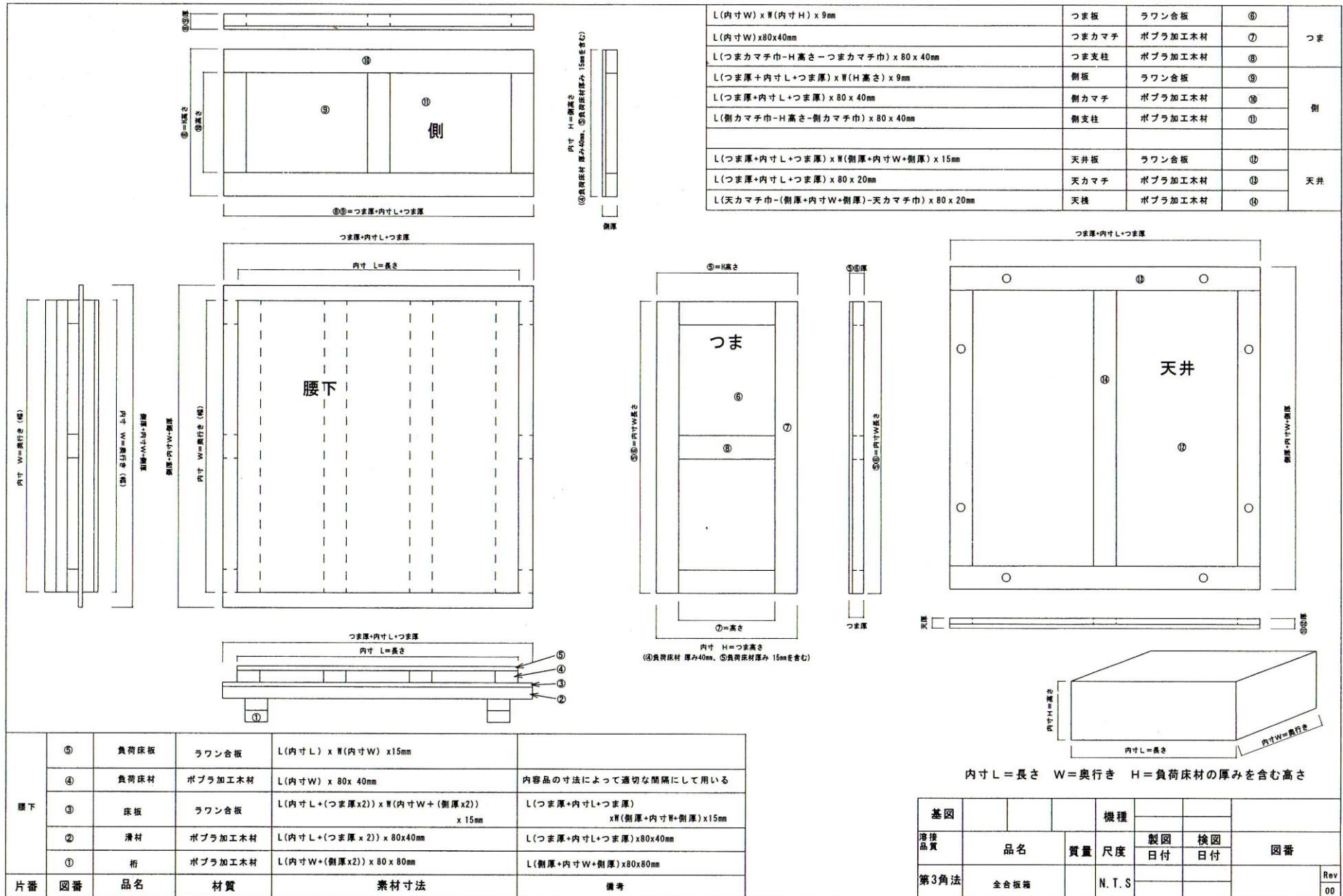
図 1—構造 (一例)
