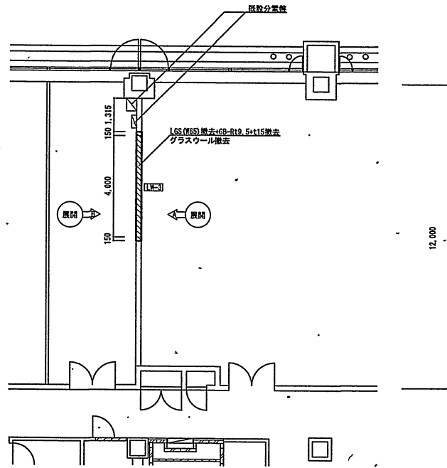
事務室②建築（床関連）平面図（整備前）
