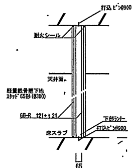
軽量鉄骨間仕切壁標準詳細図 (室内遮音壁) LW-2
