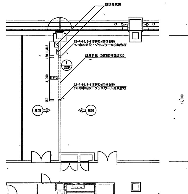
事務室②建築（床関連）平面図（整備後）
