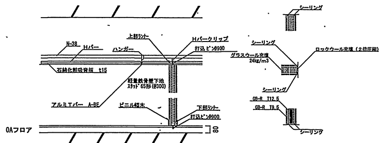
軽量鉄骨間仕切壁標準詳細図 (室内遮音壁) LW-3
