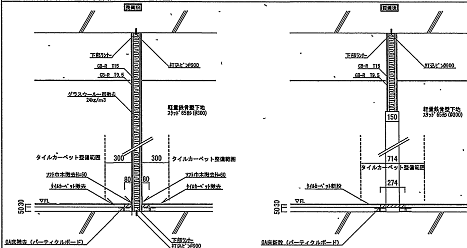
軽量鉄骨間仕切壁標準詳細図 (室内遮音壁) LW-3
