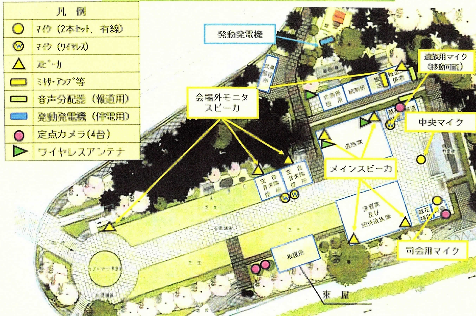
図 1ー放送設備 (晴・雨天時、メモリアルゾーン) 全般配置図
