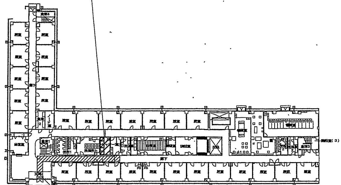
隊舎A棟1階平面図 S=1:600
