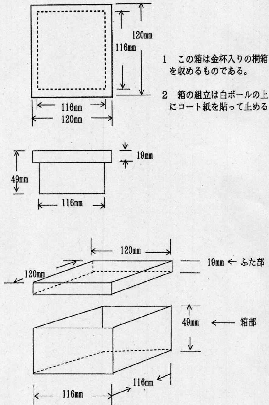
図3 包装箱 形状及び寸法(許容差±2%)
