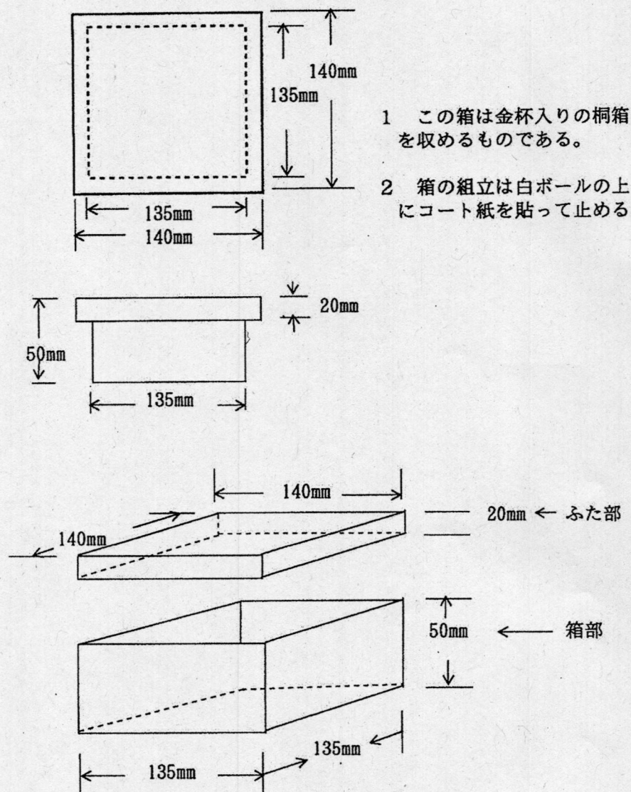
図3 包装箱 形状及び寸法(許容差±3%)
