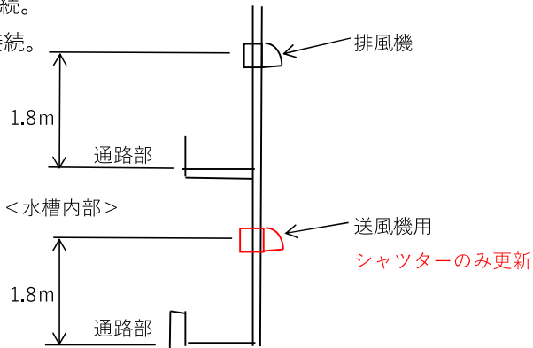
断面概要図
