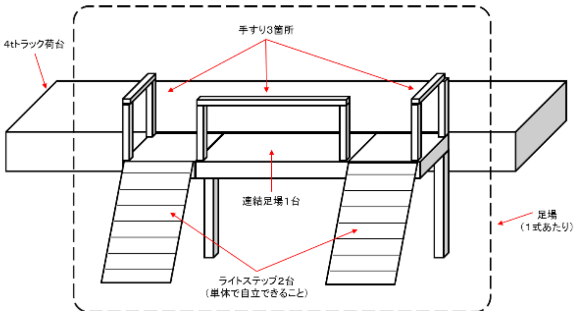
付図2 足場概要
