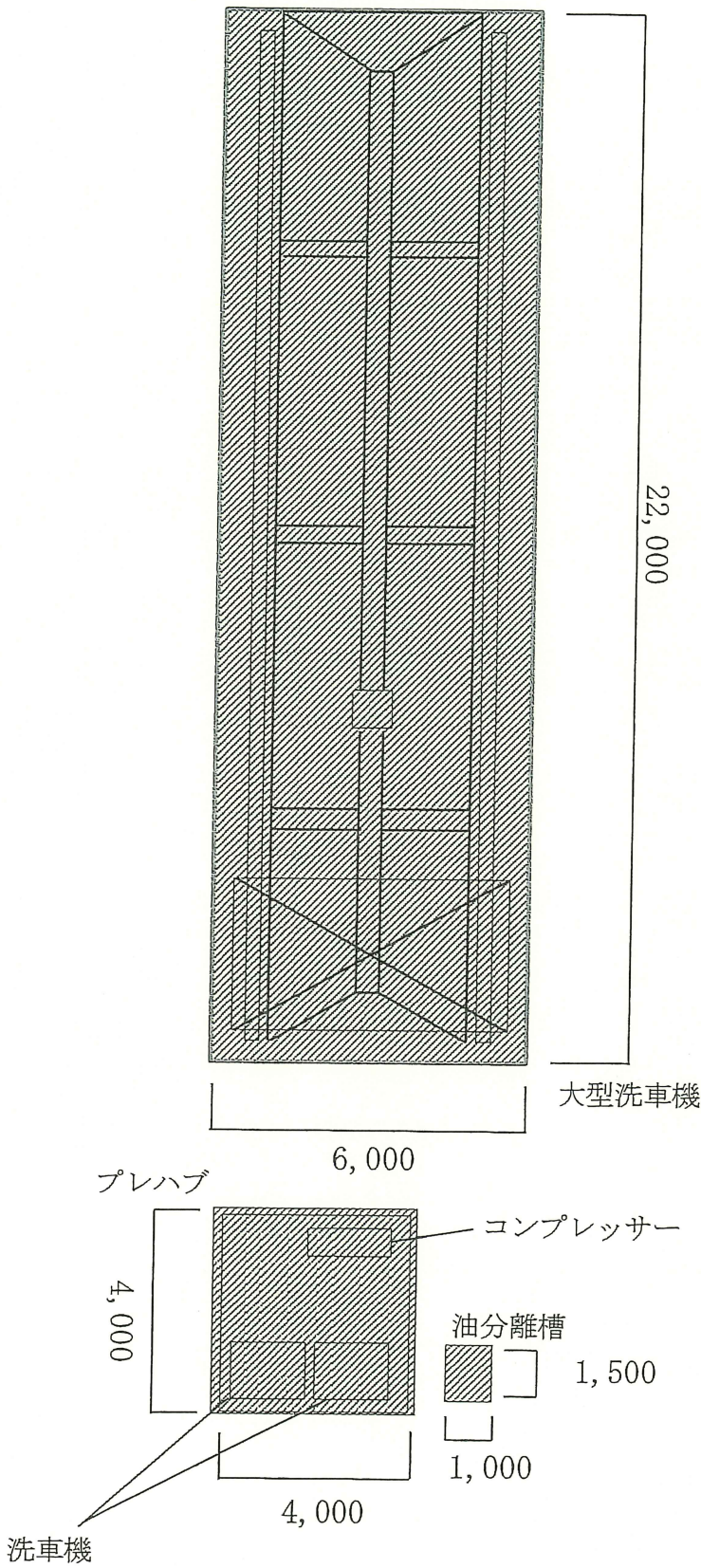
別図3 一解体範囲 (単位mm)
