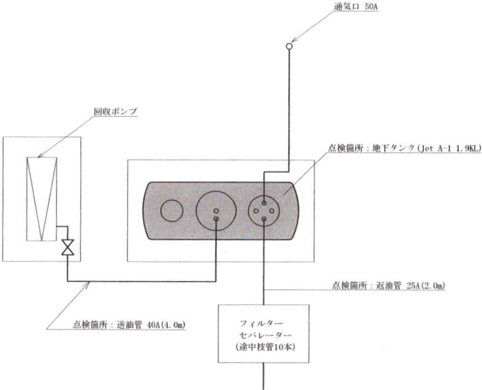
地下タンク貯蔵所H及び埋設配管図
