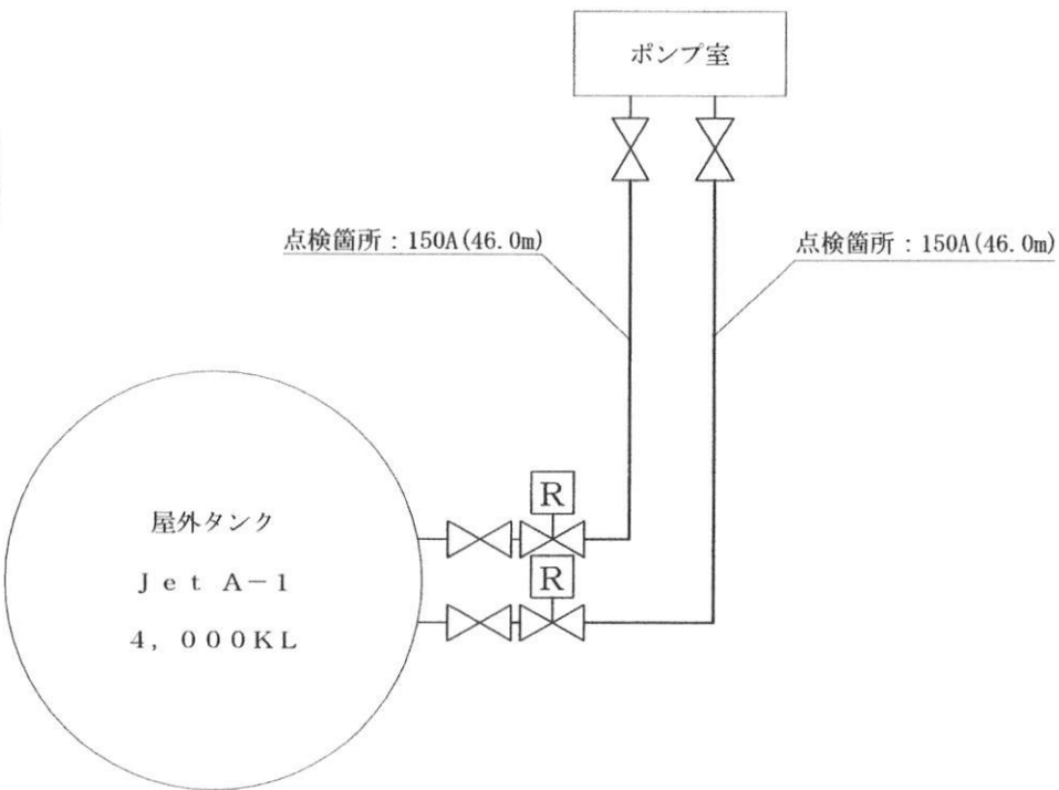
屋外タンク貯蔵所D及び埋設配管図
