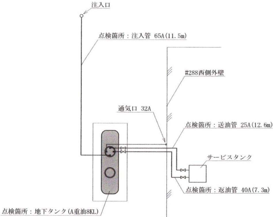
地下タンク貯蔵所D及び埋設配管図
