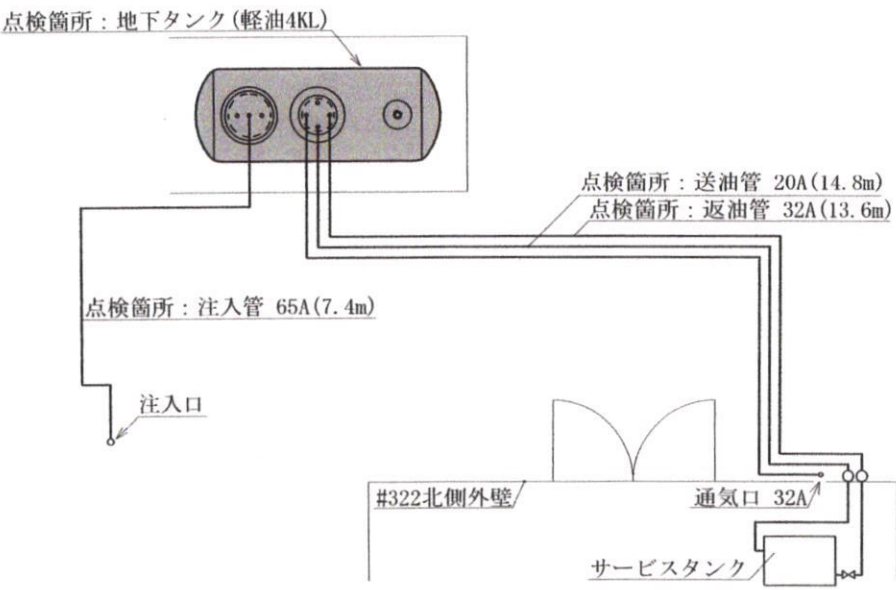
地下タンク貯蔵所C及び埋設配管図
