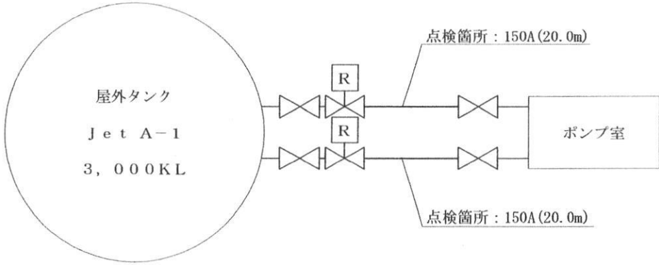
屋外タンク貯蔵所B及び埋設配管図
