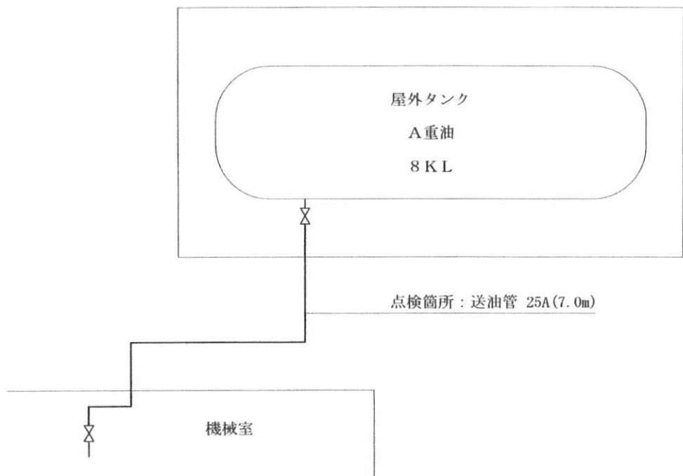
屋外タンク貯蔵所E及び埋設配管図
