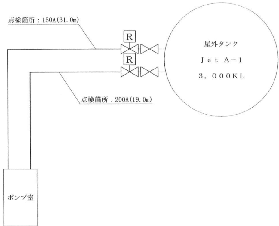
屋外タンク貯蔵所C及び埋設配管図
