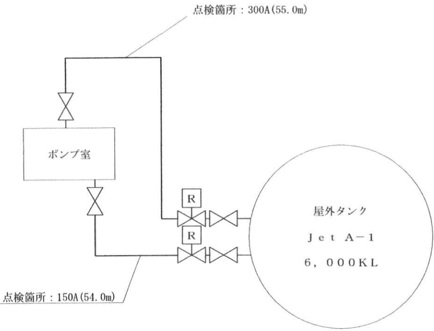
屋外タンク貯蔵所A及び埋設配管図
