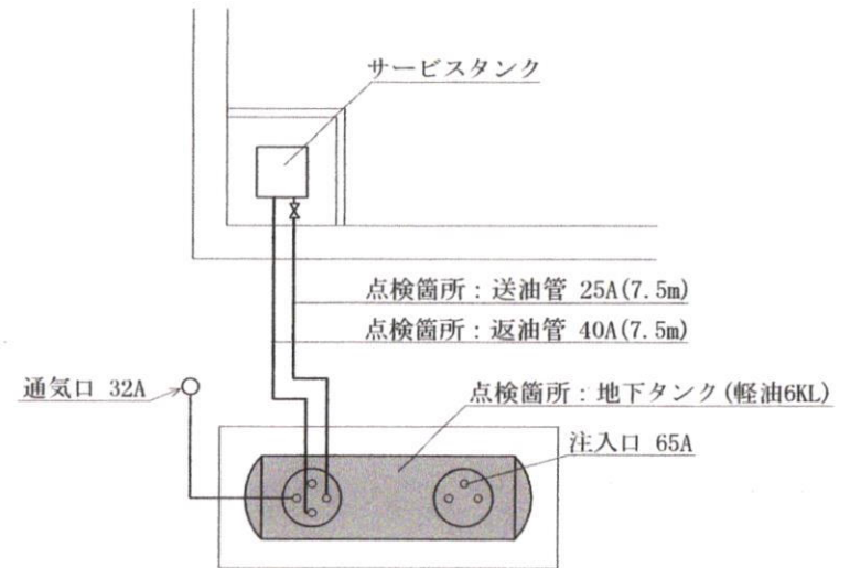
地下タンク貯蔵所F及び埋設配管図
