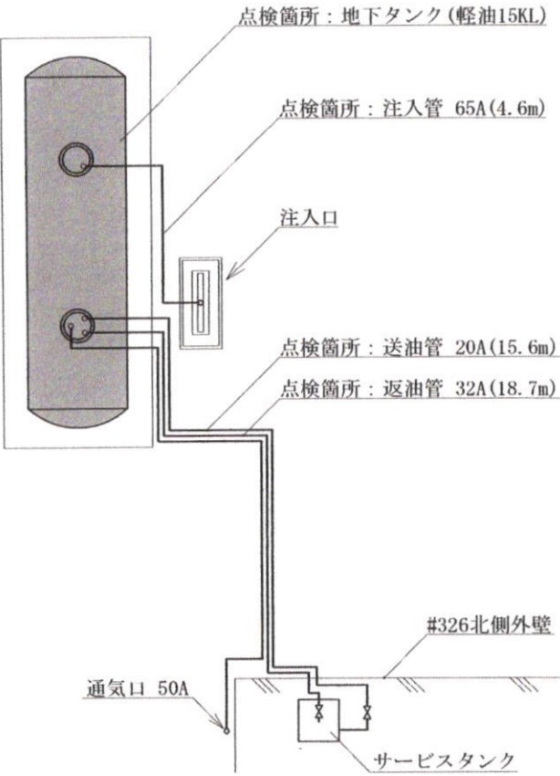
地下タンク貯蔵所G及び埋設配管図
