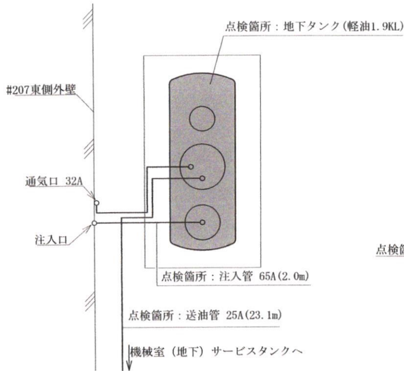
地下タンク貯蔵所A及び埋設配管図
