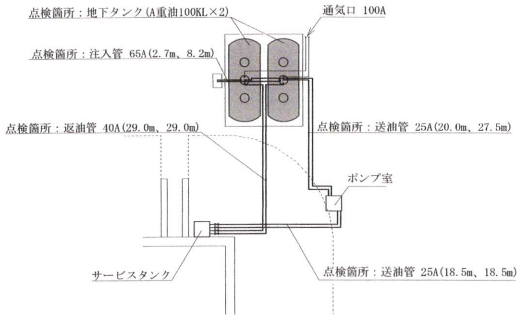
地下タンク貯蔵所E及び埋設配管図
