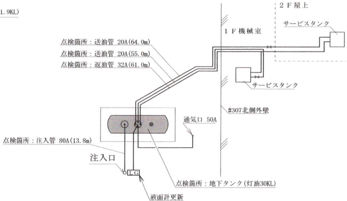
地下タンク貯蔵所B及び埋設配管図
