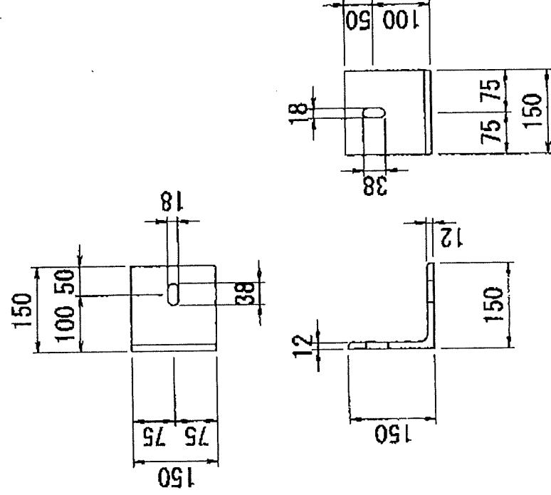
付図3 形状および寸法詳細図
