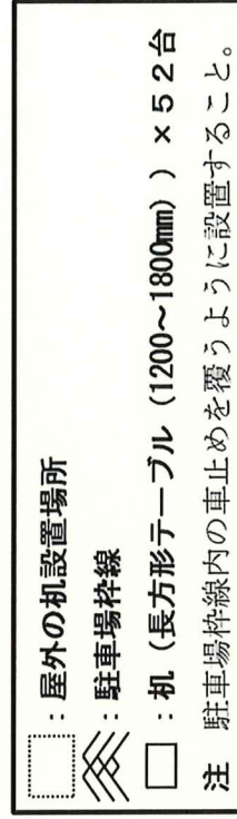
詳図 2 - 屋外の机設置場所全体
