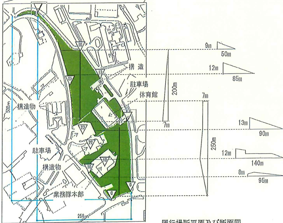
図7-履行場所細部 (業務隊本部周辺及び体育館周辺)
