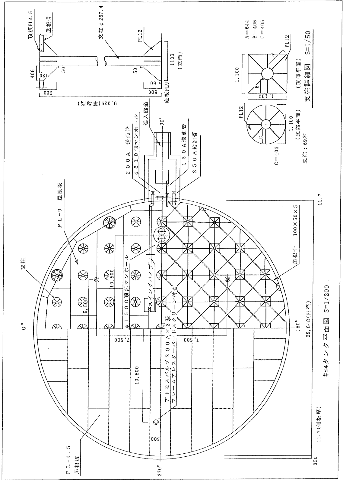
図2-1平面図
