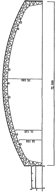
断面図 S=N/S
