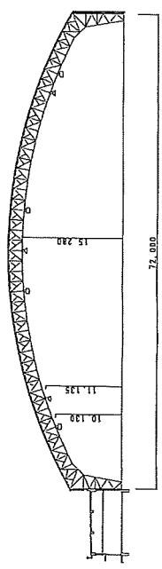
断面図 S=N/S
