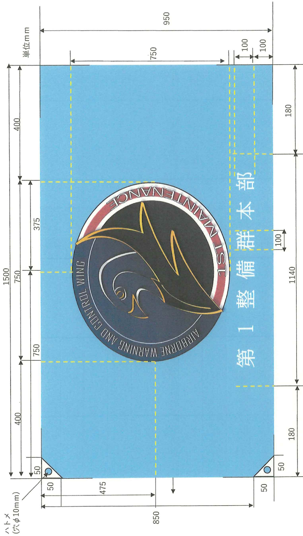
注記1 「第1整備群本部」はBIZ UD明朝 Mediumとし、大きさは1140mmに収まる範囲とする。
