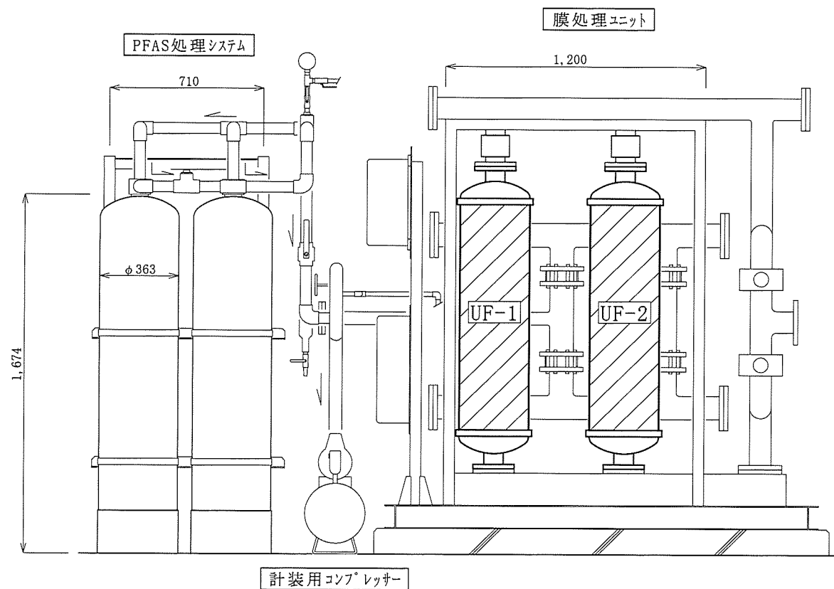
A - A 立面図
