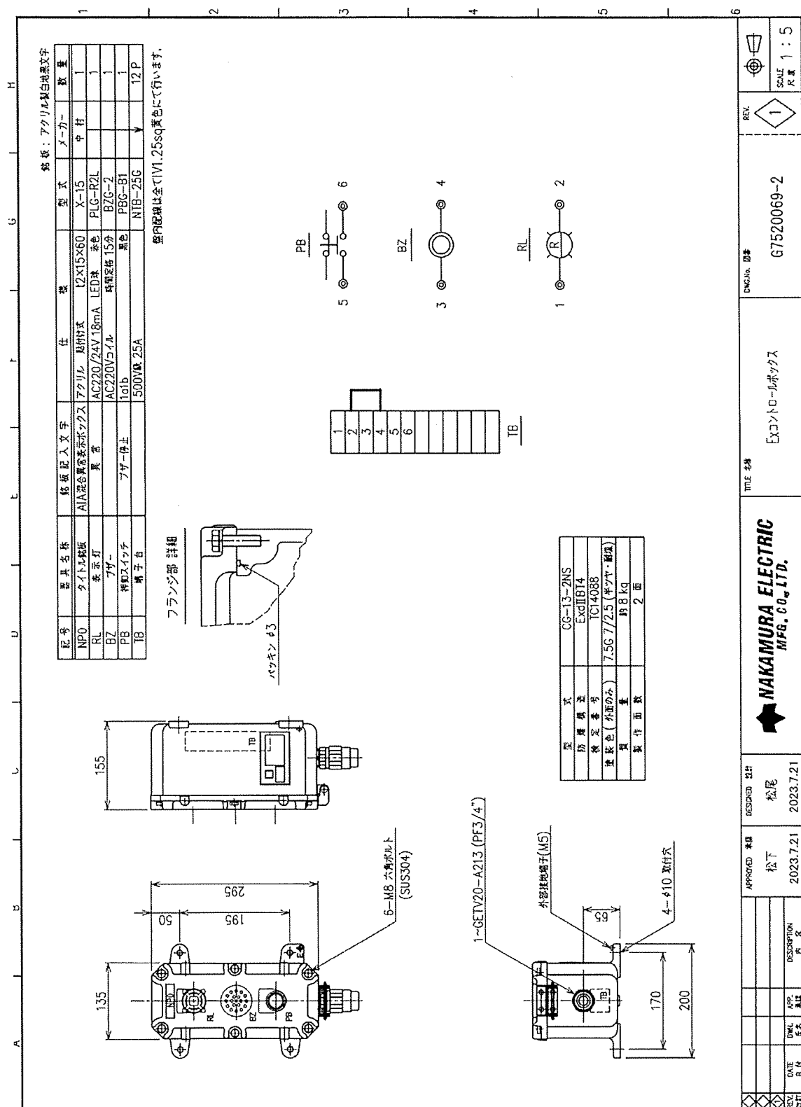
A I A混合異常表示ボックス外観図
