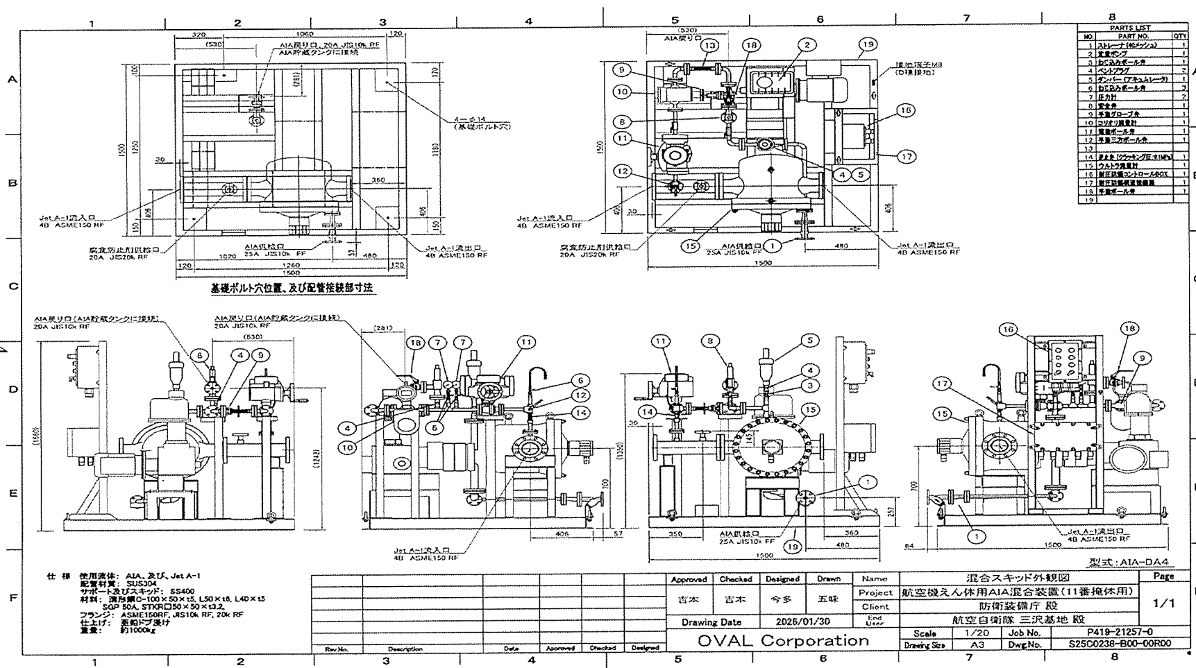
11番掩体A I A混合装置外観図
