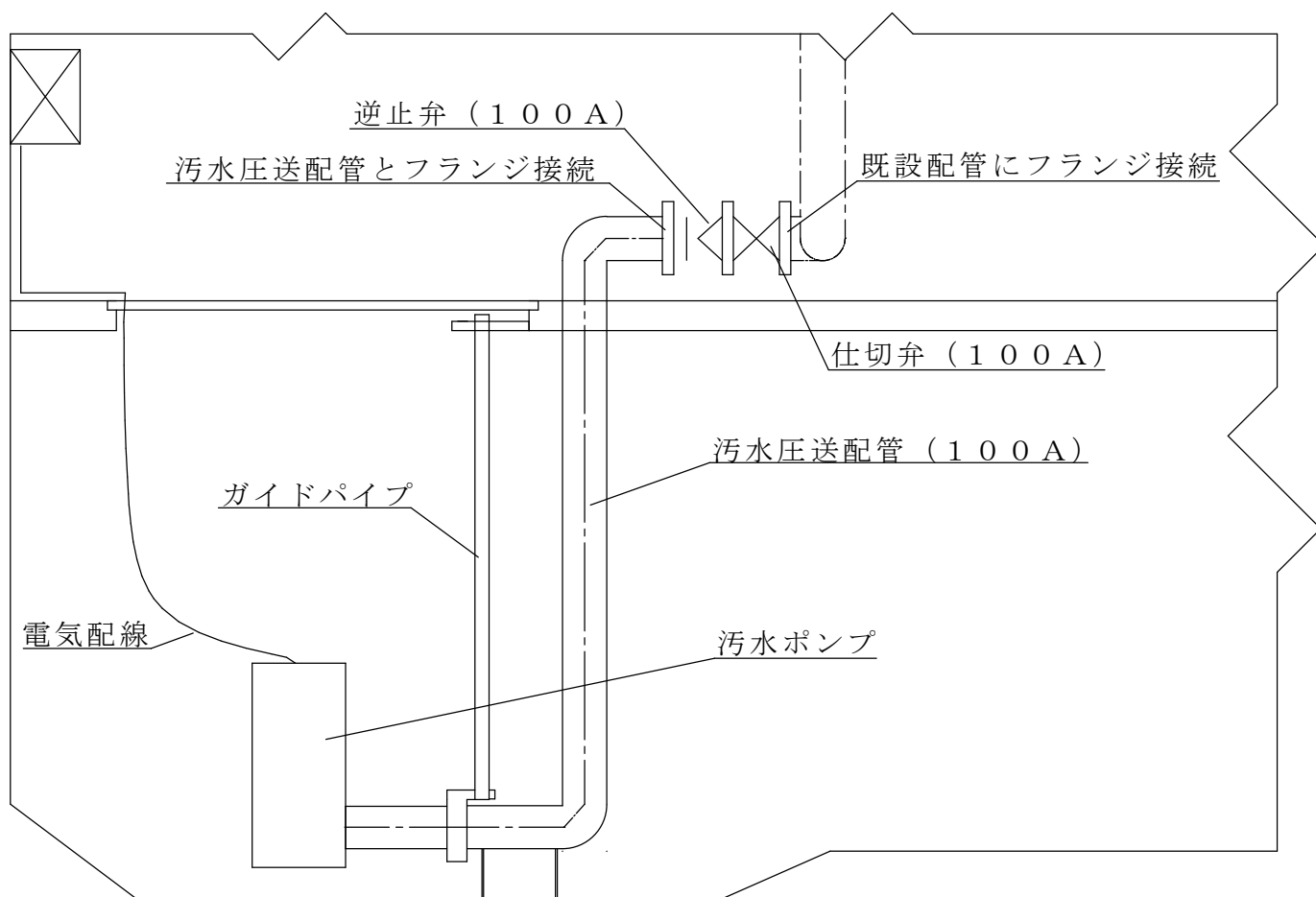
# 1 2 8 補修箇所断面図 (NONE SCALE)
