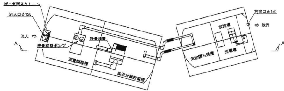
内部平面図
