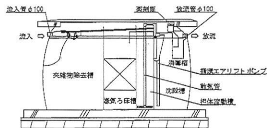
A-A' 断面図
