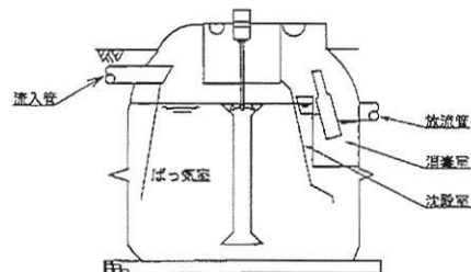
A-A' 断面図
