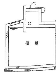
A-A' 断面図
