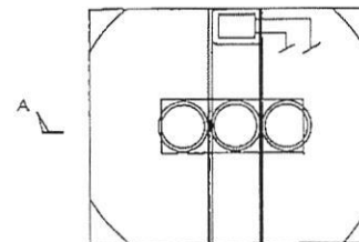
内部平面図
