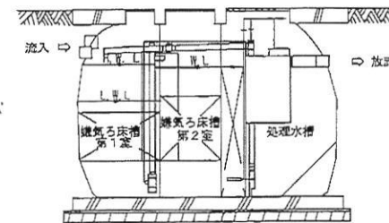
A-A' 断面図
