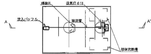
内部平面図
