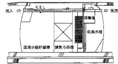
A-A' 断面図
