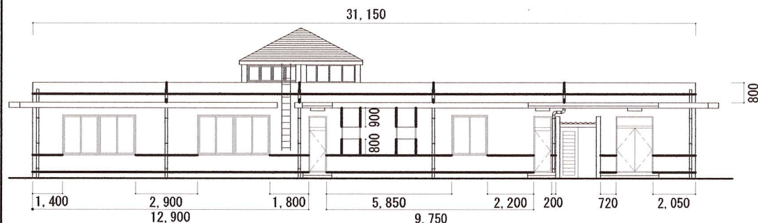
D面立面図 1/250
