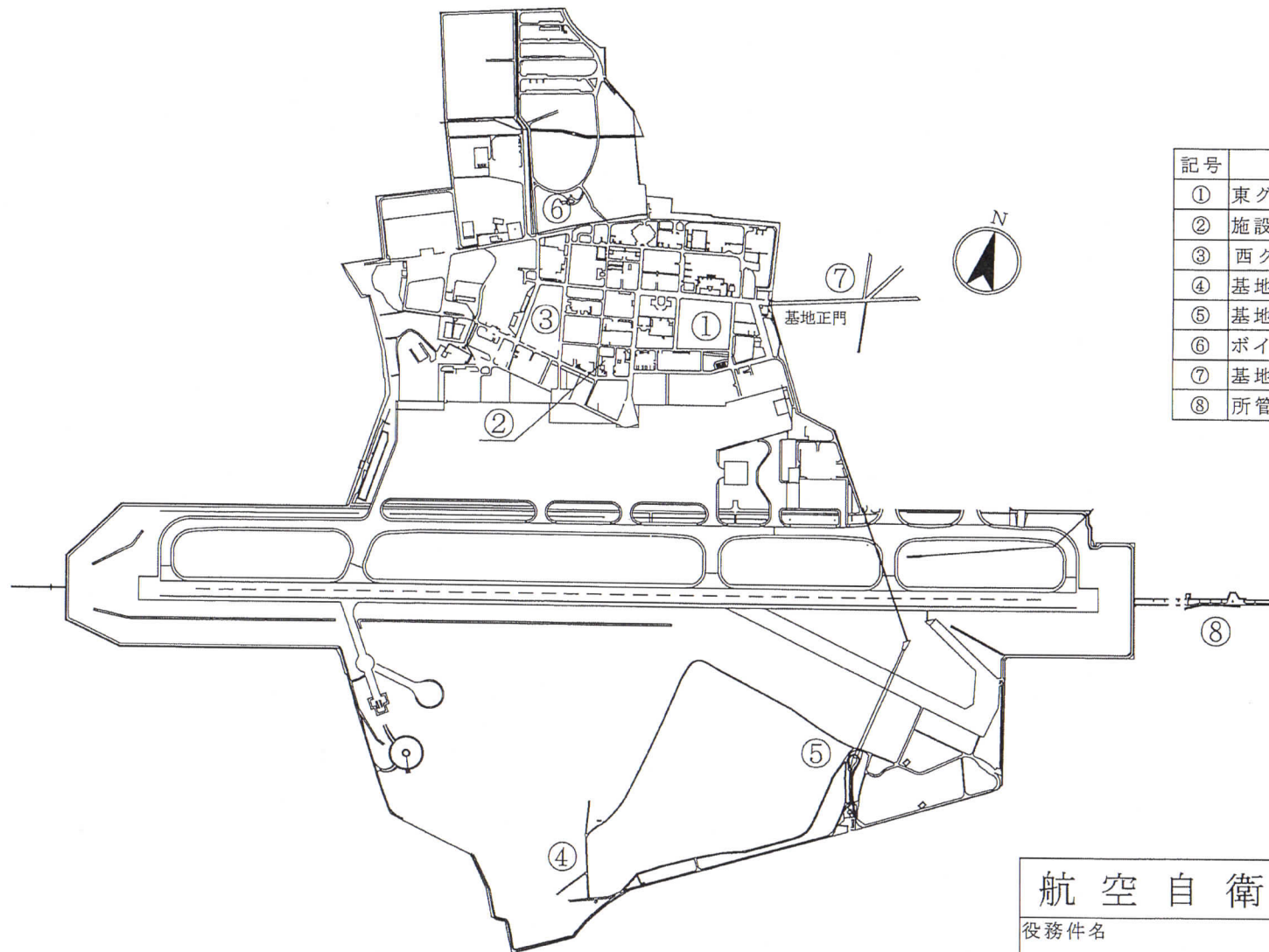
基地全体図
