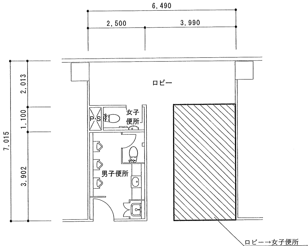
4 階女子便所詳細図 1/100
