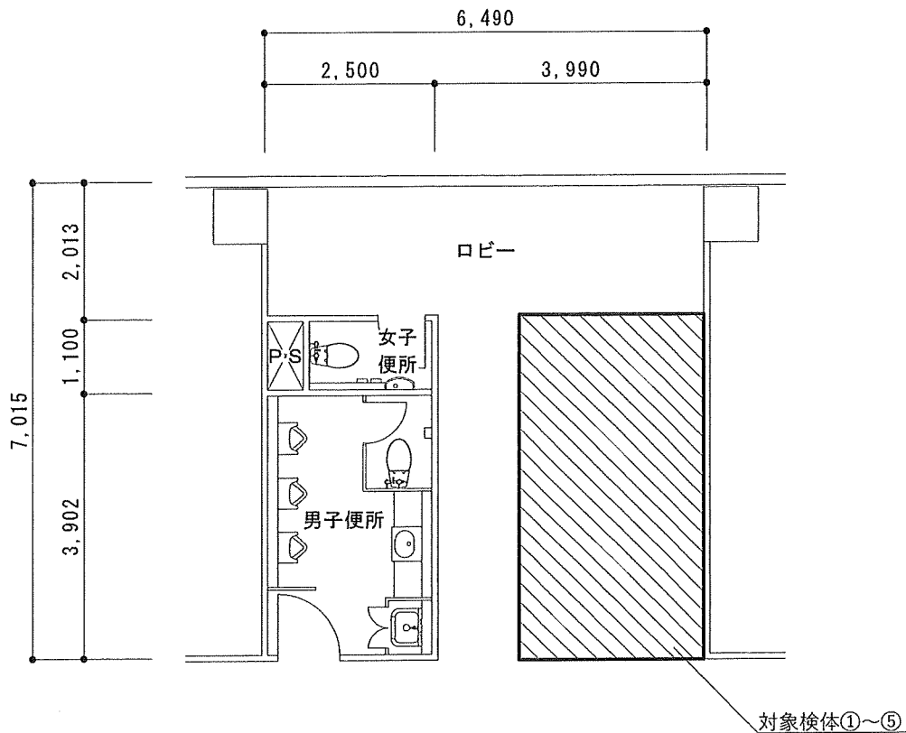
4階女子便所詳細図 1/100
