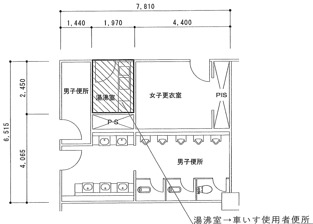
3階車いす使用者便所詳細図 1/100
