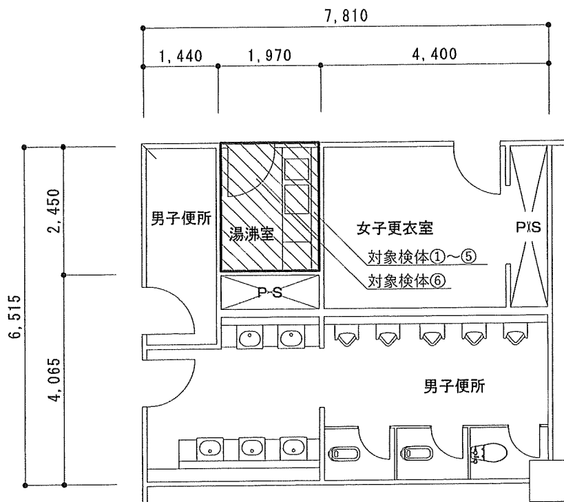
3階車いす使用者便所詳細図 1/100
