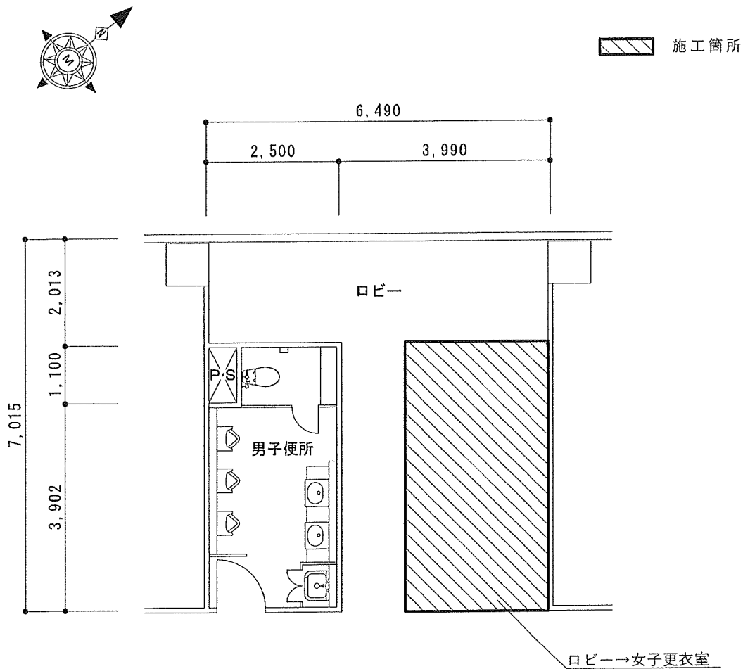
3 階女子更衣室詳細図 1/100
