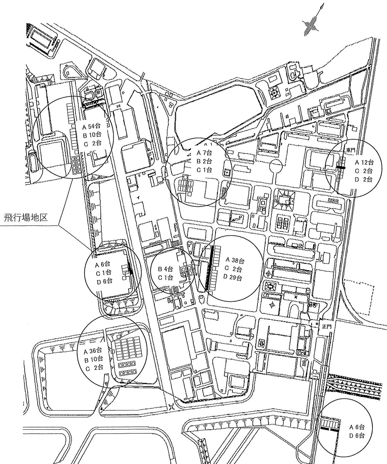
借上仮設トイレの規格及び数量表(別図第2を含む)
