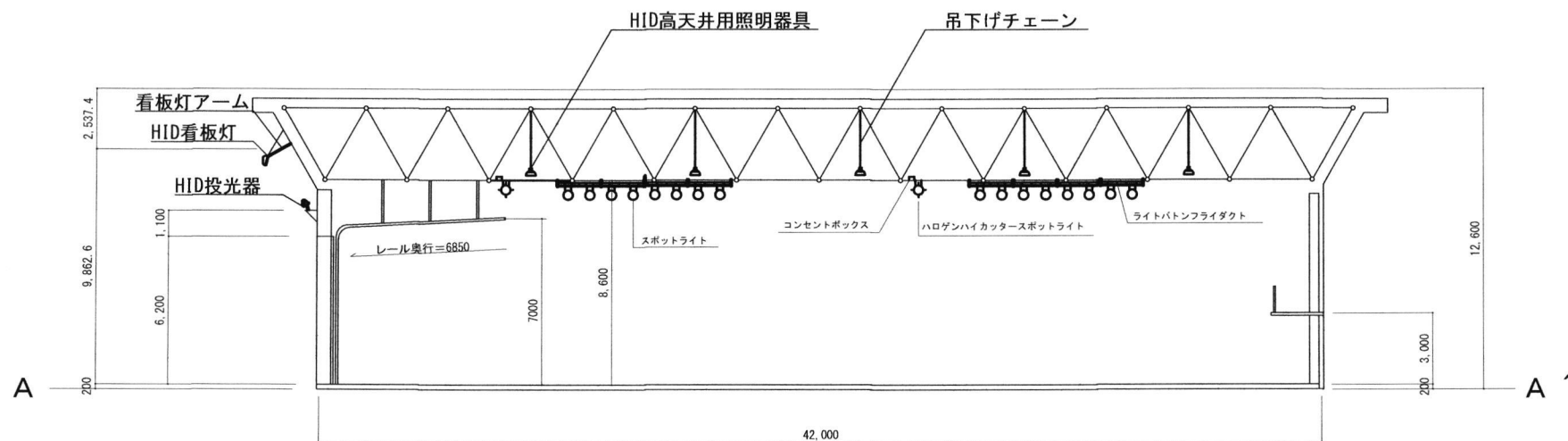
A - A' 断面図 (撤去)
