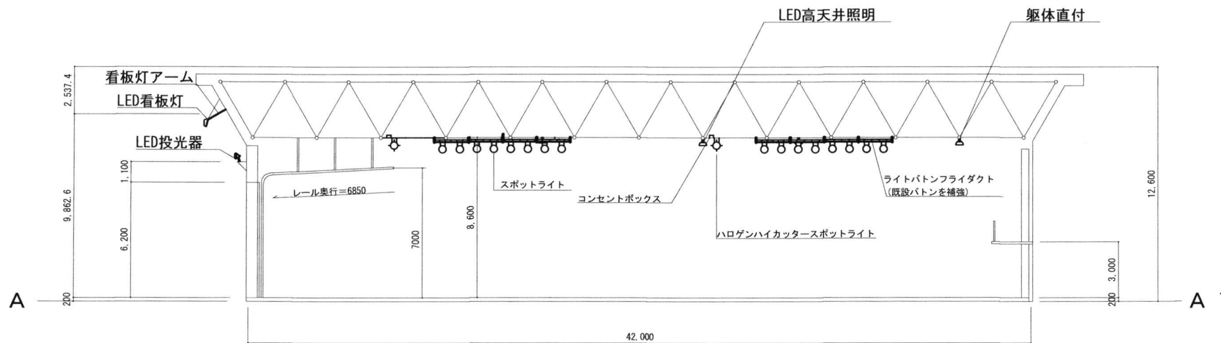
A - A' 断面図 (新設)
