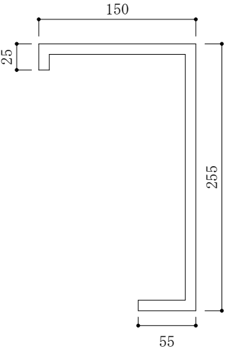
笠木断面図
