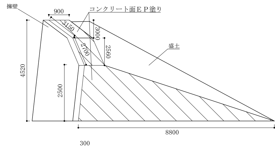
擁壁立面図 S = 1 / 1 0 0
