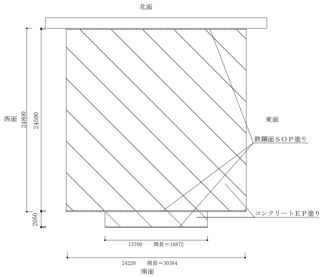
平面図 S = 1 / 3 0 0
