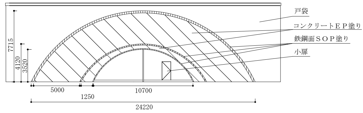
南面立面図（詳細図） S = 1 / 2 5 0
