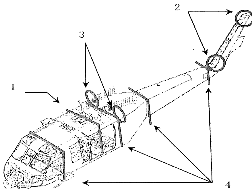
図一用廃機の解体要領
