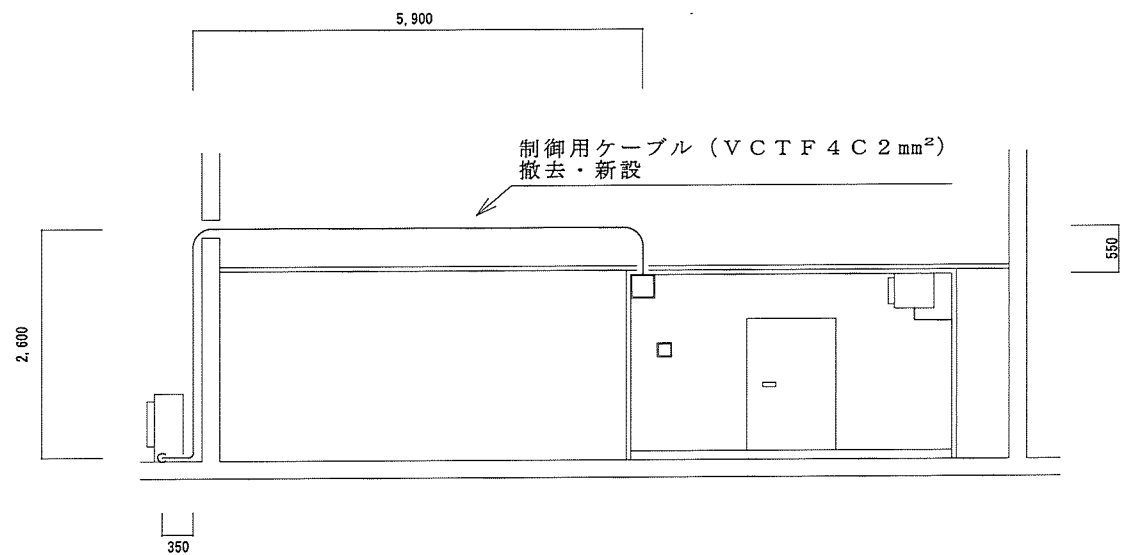
立面図
