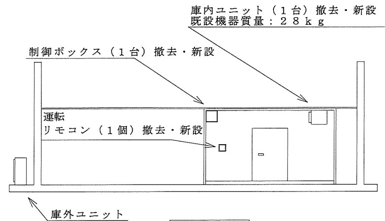
立面図
