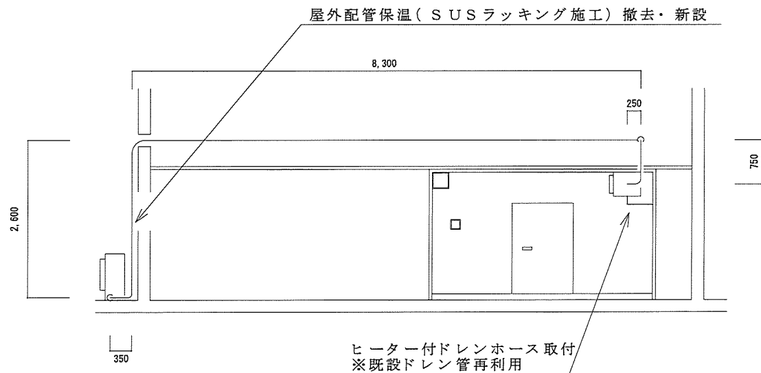
立面図
