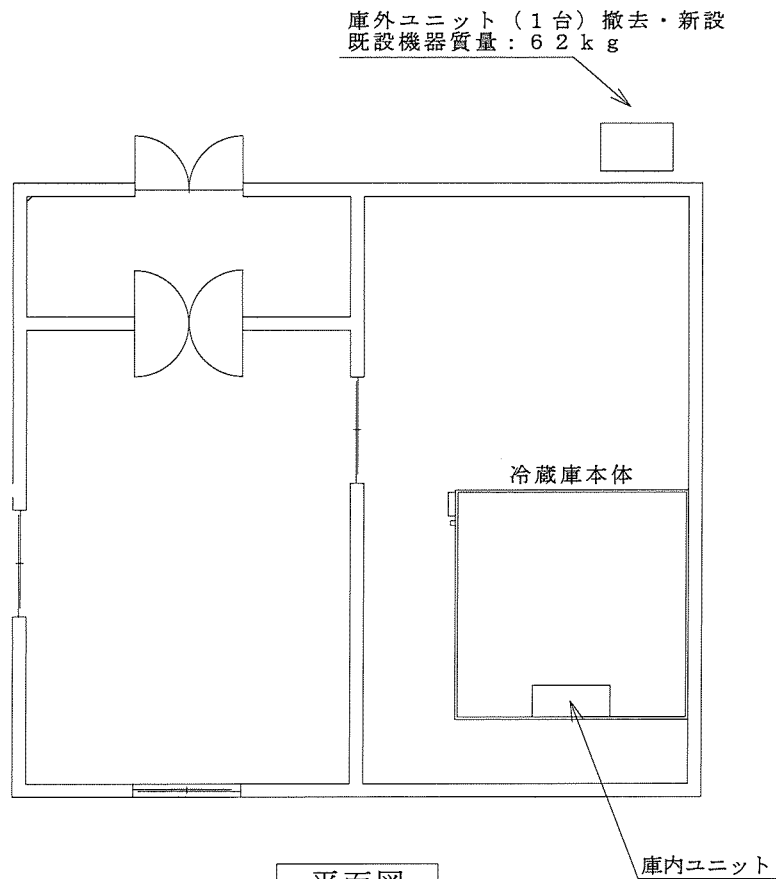
平面図
