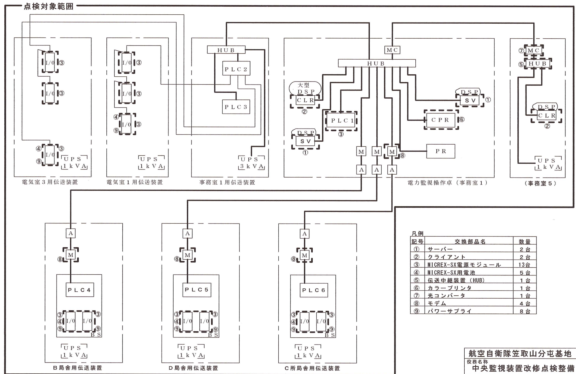
付図 3 : 中央監視装置構成図
