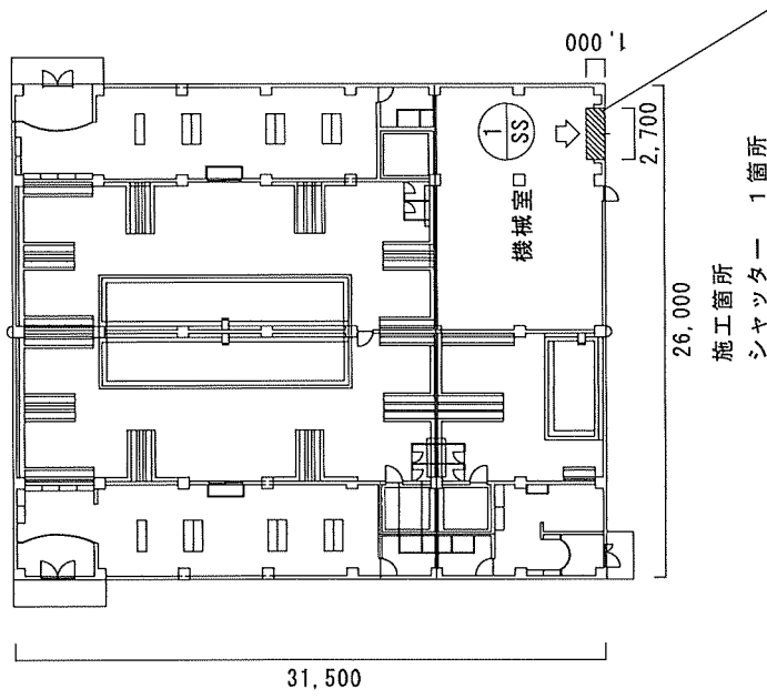
基地浴場平面図 S=1/300
