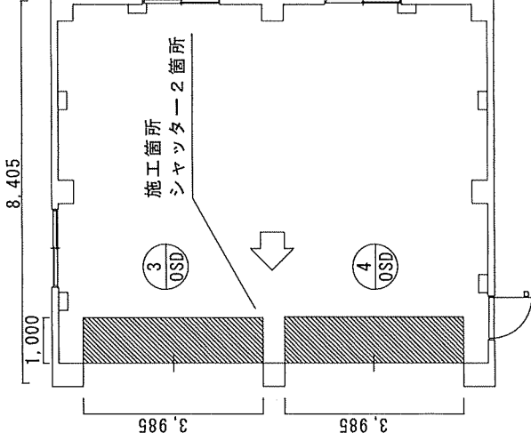
救急車庫 平面図 S=1/100
