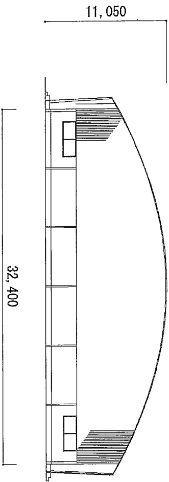
C 立面图
